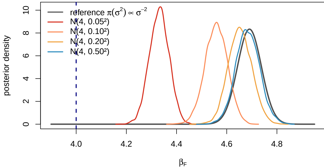
Posterior of \beta_F vs prior strength
