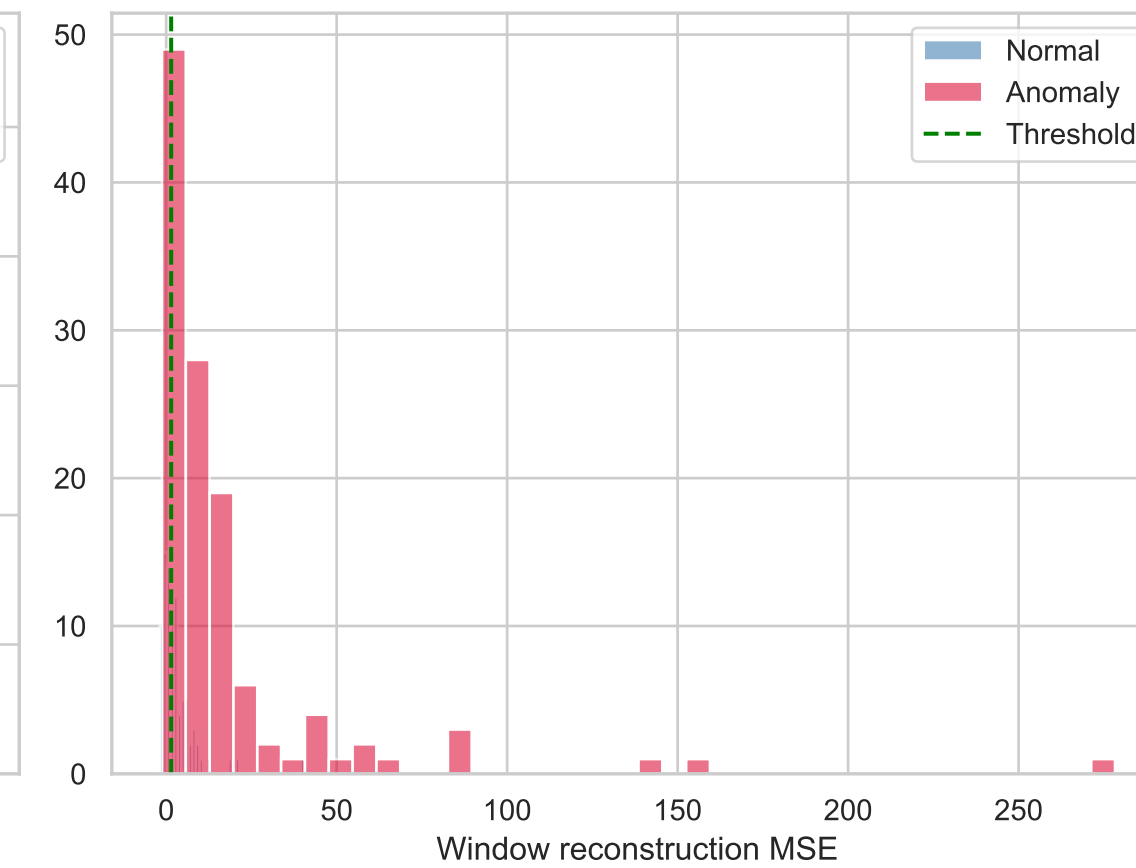
LSTM autoencoder error
