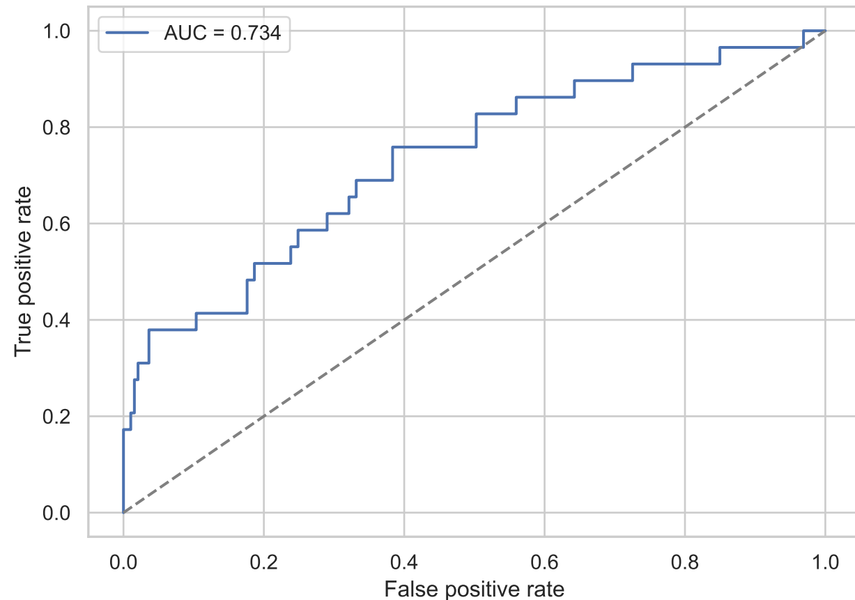
ROC - Grouped COPOD
