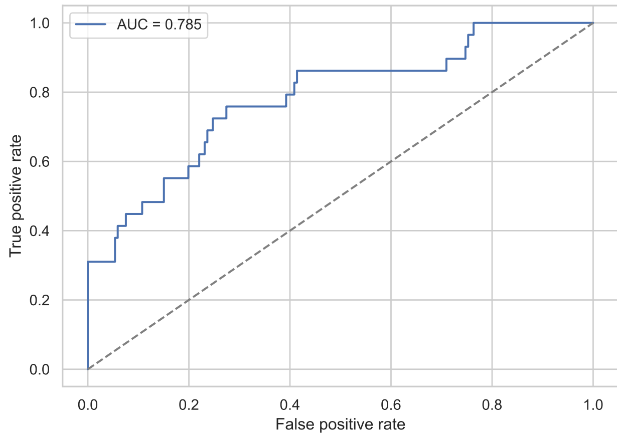
ROC - LSTM autoencoder
