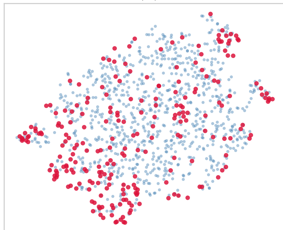
VAE latent (mu) -- t-SNE
