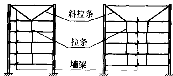
图 8.4.2 拉条布置示意图
