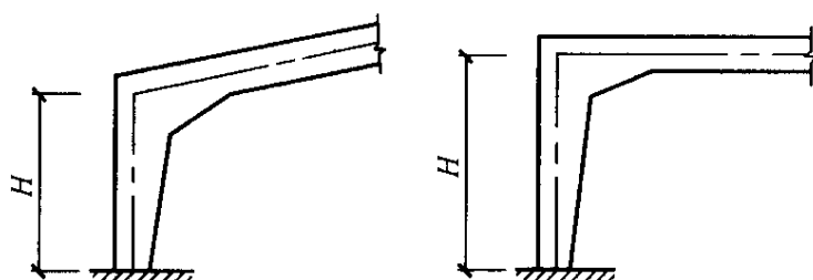
图 10.1.2 刚架柱的高度示意图
