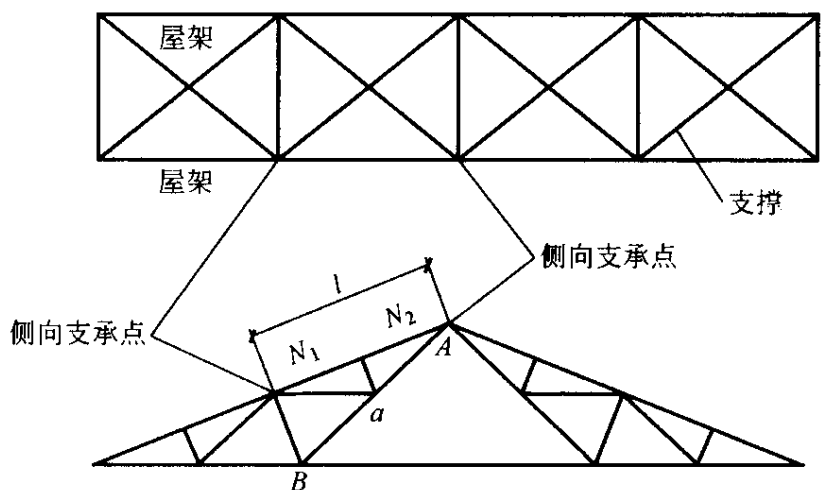
图 9.1.2 屋架杆件计算长度示意图
