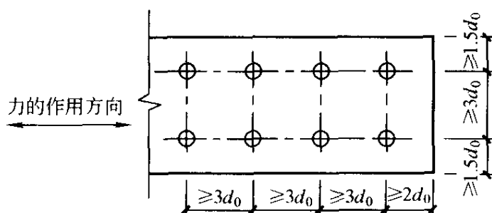
图 6.2.4 螺栓最小间距示意图
