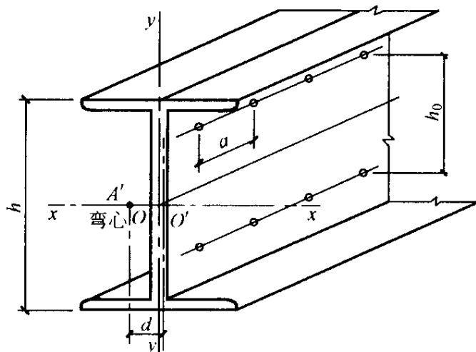
图 6.1.8 组合工形截面示意图
