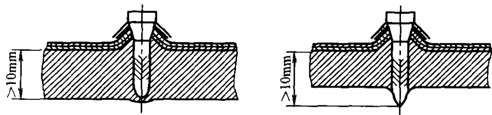
图 6.2.8 射钉的穿透深度
