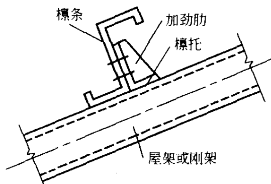
图 8.2.1 实腹式檩条端部连接示意图
