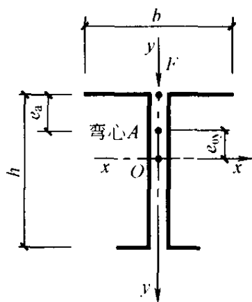
图 A. 2. 2 单轴对称截面示意图
