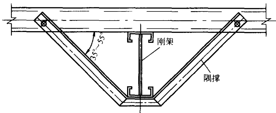
图 10.2.4 刚架梁或柱的隅撑
