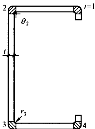
图 C.0.1 冷弯薄壁型钢截面示意图
