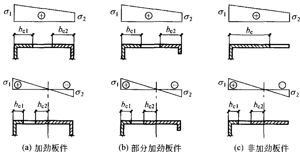
图 5.6.5 受压板件的有效截面图
