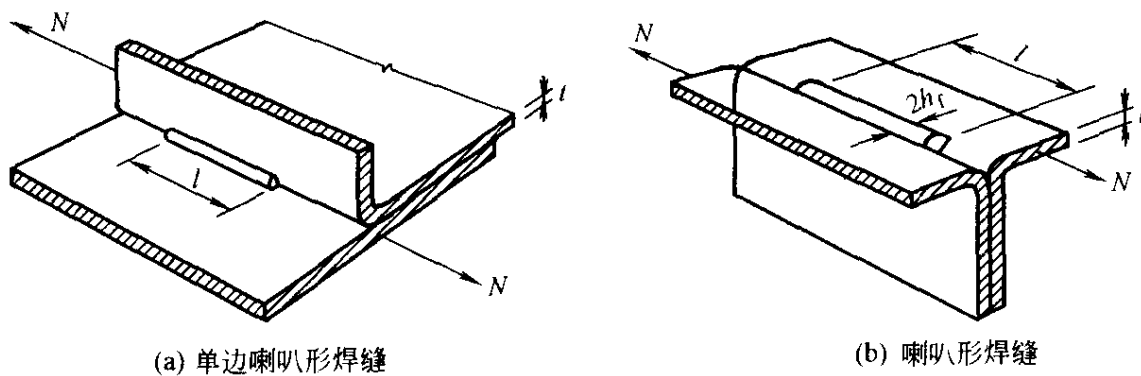
图 6.1.2-2 纵向受剪的喇叭形焊缝
