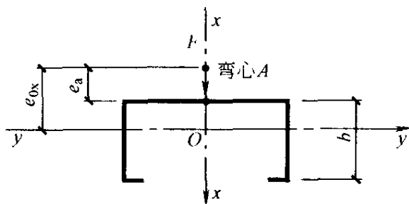
图 A. 2. 3 单轴对称卷边槽钢
