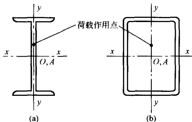
图 5.5.2 双轴对称截面示意图
