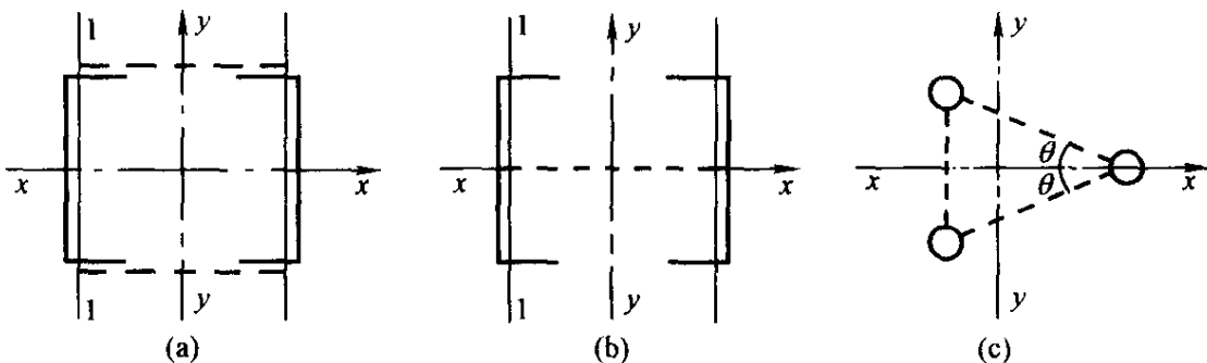
图 5.2.6 格构式构件截面示意图
