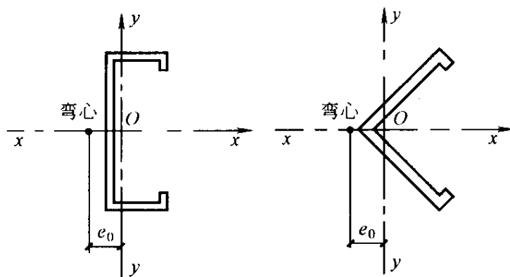
图 5.2.4 单轴对称开口截面示意图
