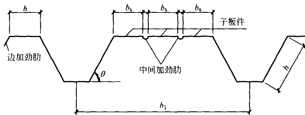
图 7.1.2 压型钢板截面示意图
