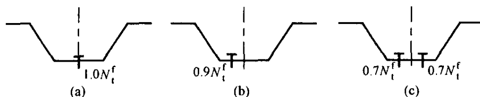
图 6.1.7 压型钢板连接示意图
