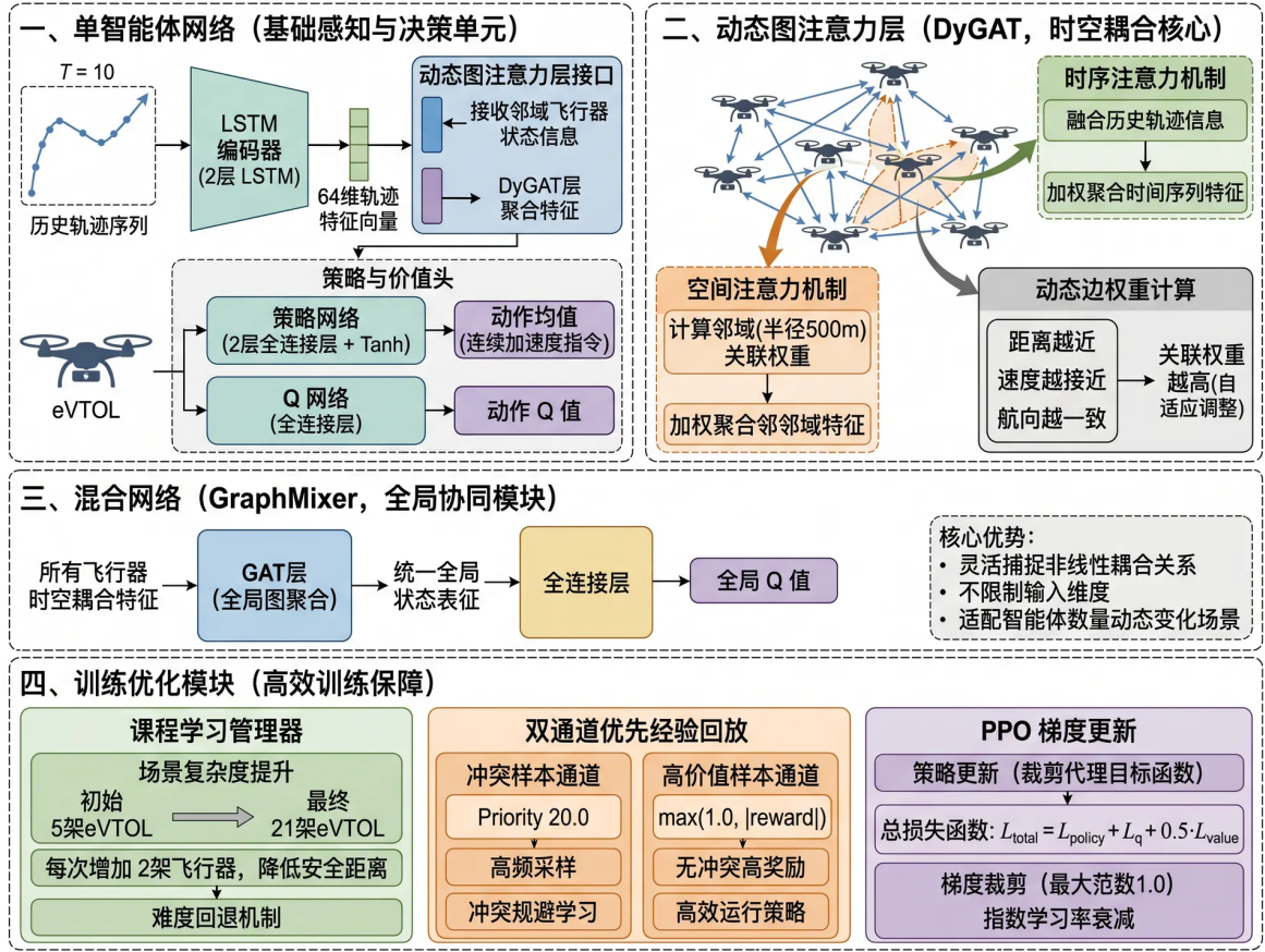
图 1: 模型整体架构——环境层、编码层 (LSTM+DyGAT 含乘法门控注意力掩码)、决策层 (策略头 + Q 值头 + GAT-Mixer) 与训练层 (课程学习 + 冲突损失加权 + PPO)。
