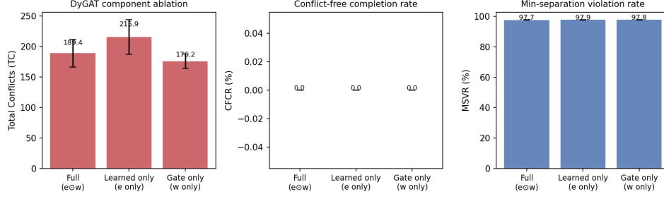
图 7: 补充组件级消融：移除门控使 TC 上升约 14%，纯门控与完整模型相当（缩小规模环境）。
