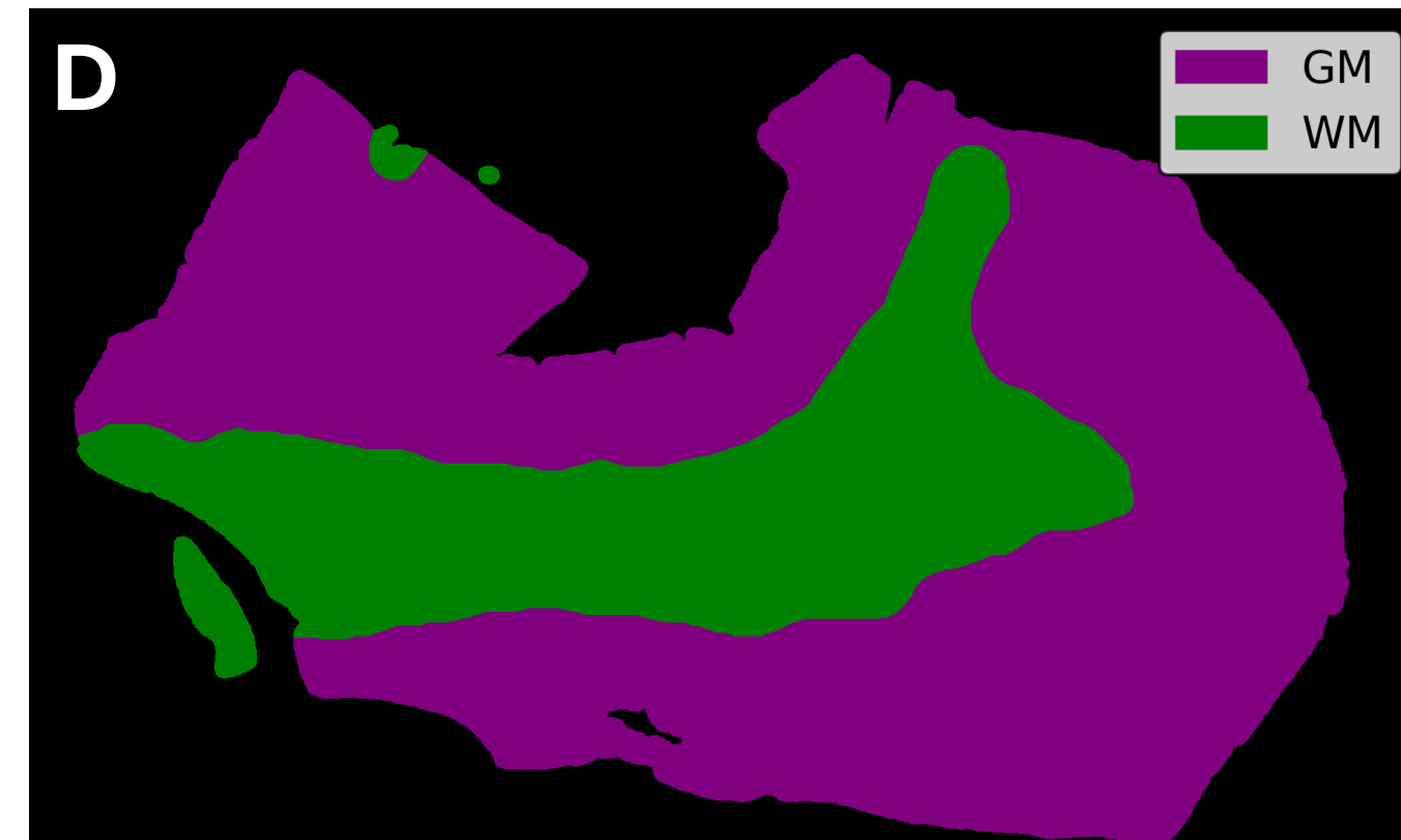
NEUSEG
