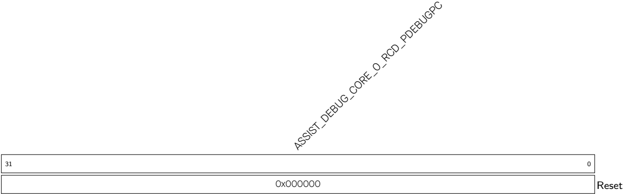
Register 17.19. ASSIST_DEBUG_CORE_O_RCD_PDEBUGPC_REG (0x0048)
