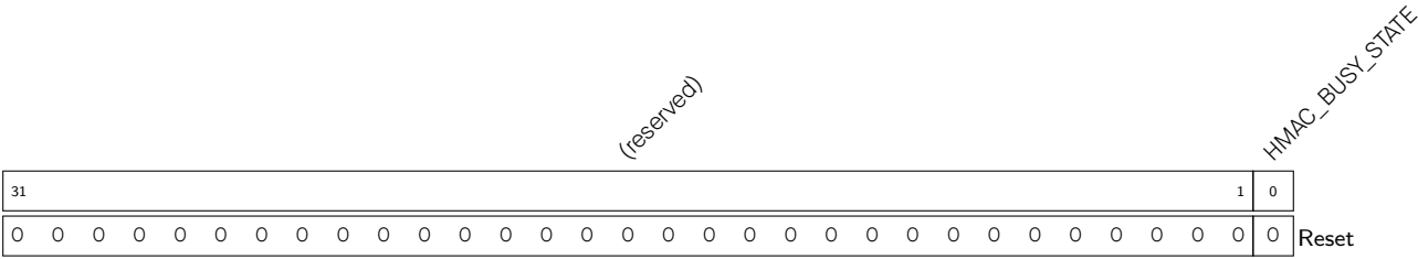
Register 19.10. HMAC_QUERY_BUSY_REG (0x006C)
