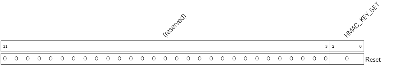
Register 19.12. HMAC_SET_PARA_KEY_REG (0x0048)
