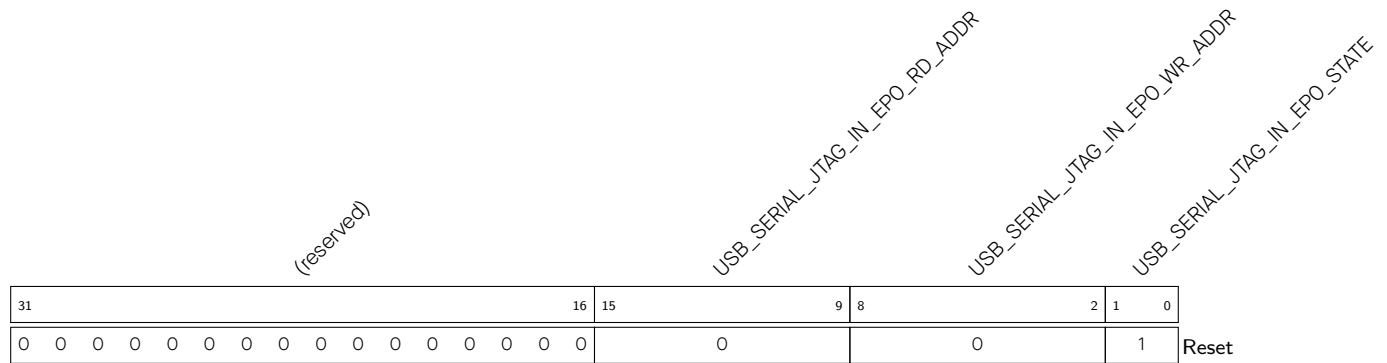
Register 30.9. USB_SERIAL_JTAG_IN_EPO_ST_REG (0x0028)
