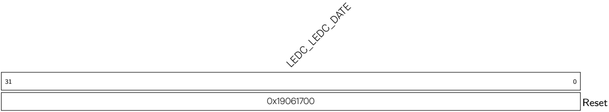
Register 32.13. LEDC_DATE_REG (0x00FC)
