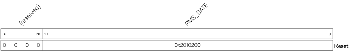
Register 14.72. PMS_DATE_REG (0x0FFC)
