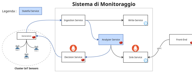
Fig. 3. Visione ad alto livello del Sistema.
