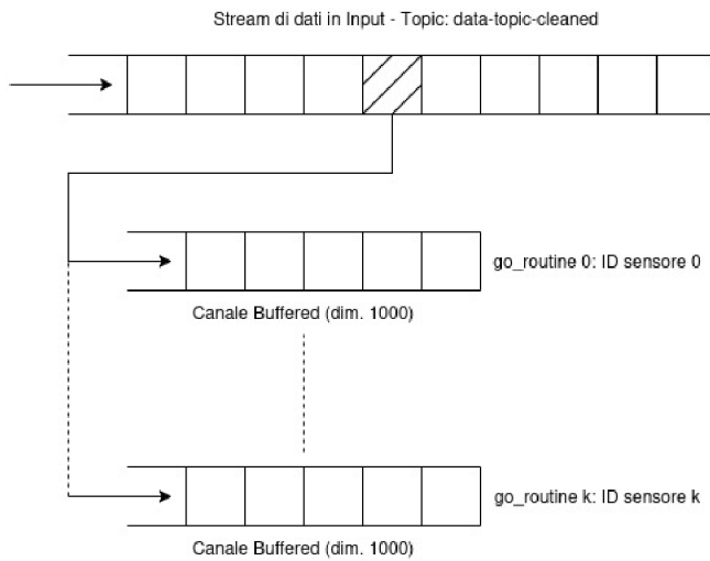
Fig. 2. Dispatcher messaggi.
