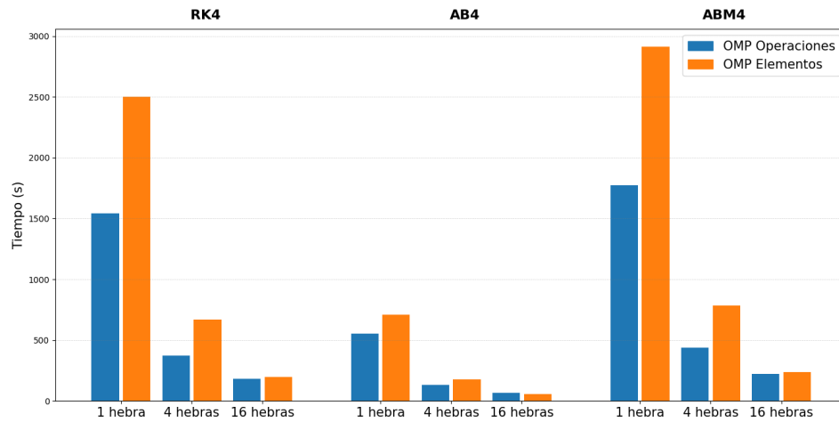
Figura 3.3: Brusselator1D 100.000 ecuaciones
