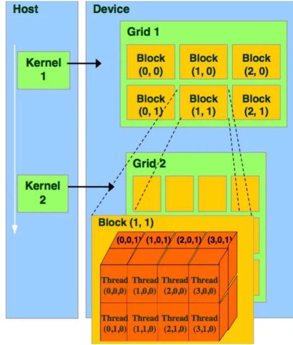
Figura 2.7: Grids y bloques CUDA [Casas, 2024]
