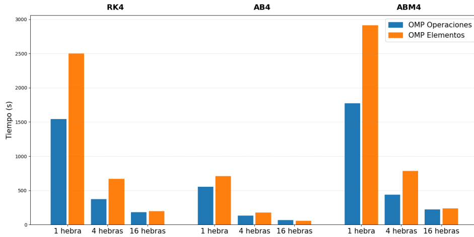
Figura 3.3: Brusselator1D 100.000 ecuaciones
