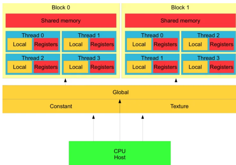
Figura 2.8: Jerarquía de memorias en CUDA [Beard, 2020]
