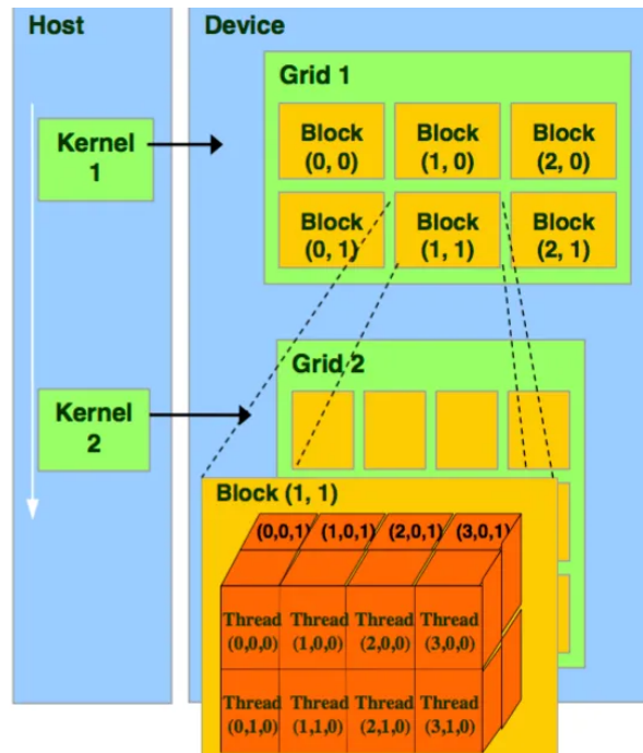
Figura 2.9: Grids y bloques CUDA [Casas, 2024]
