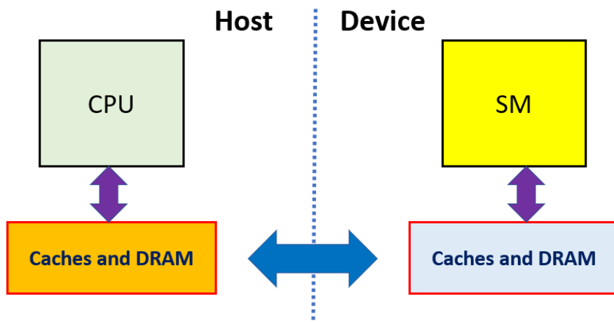
Figura 2.7: Modelo host-device de CUDA
