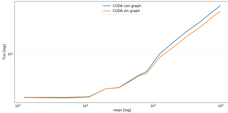
Figura 4.9: Comparación de tiempos de graph con ABM en Brusselator2D
