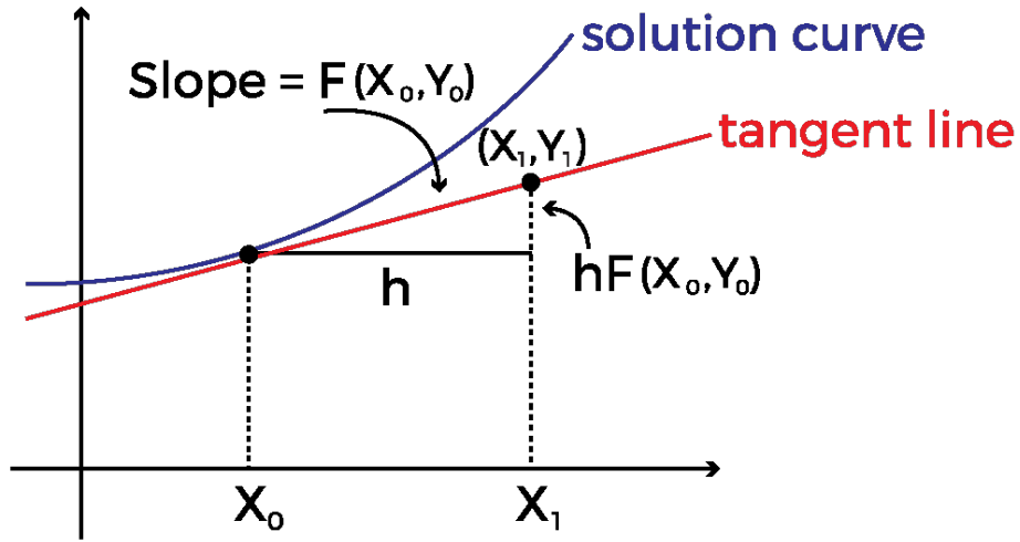
Figura 2.1: Aplicación del método de Euler
