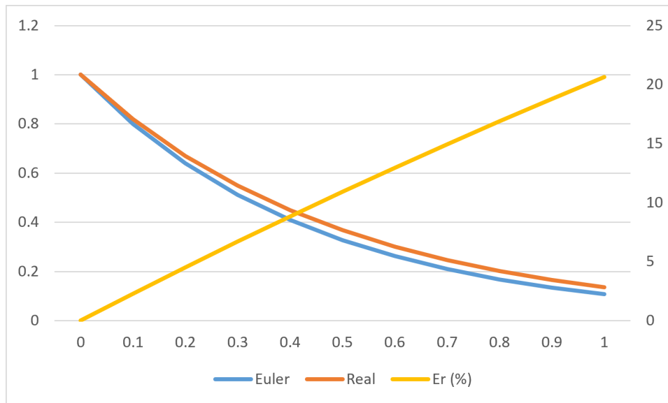
Figura 2.2: Comparativa entre Euler y valor real
