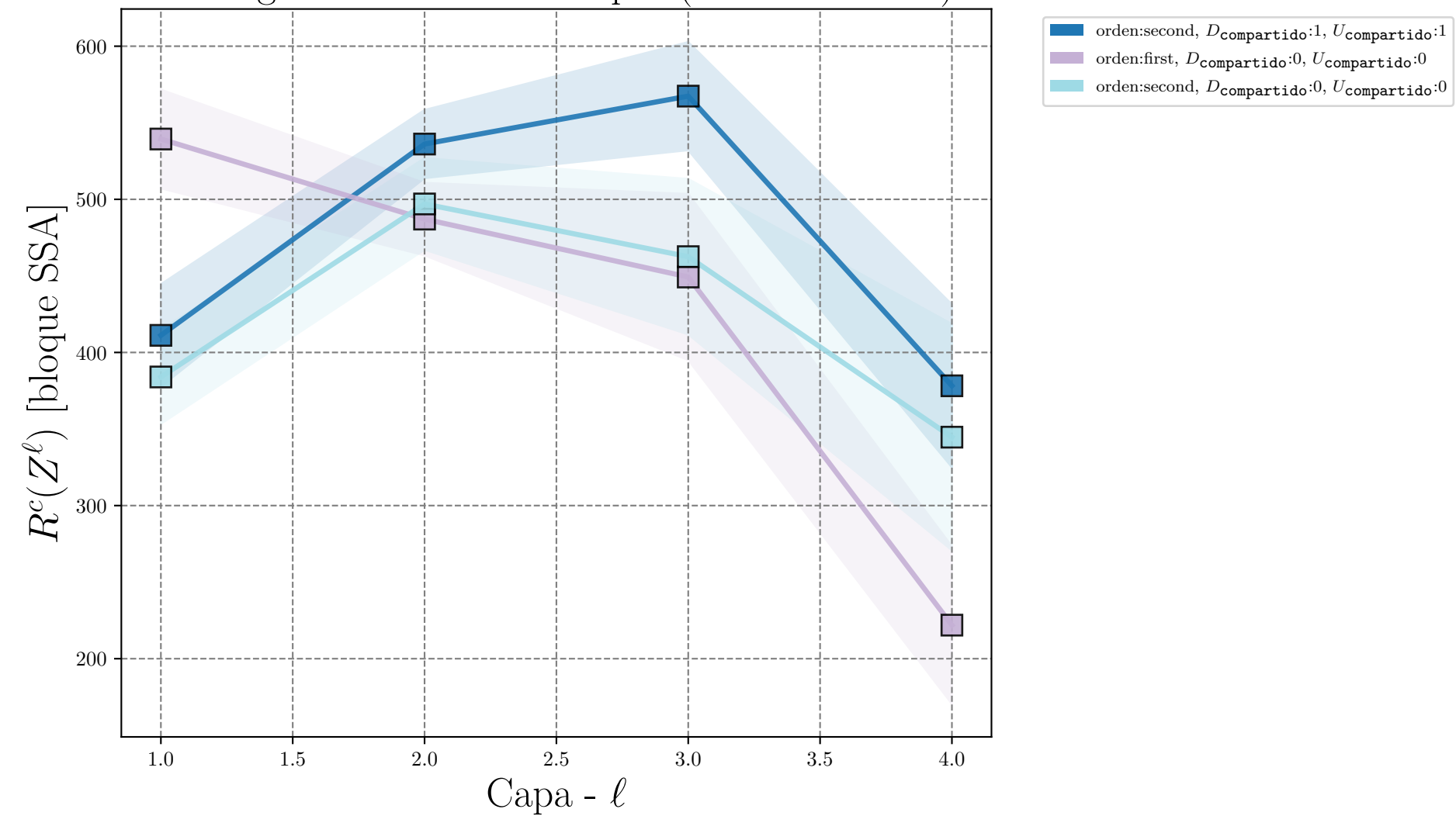
Coding Rate travesso das capas (menos é melhor)
