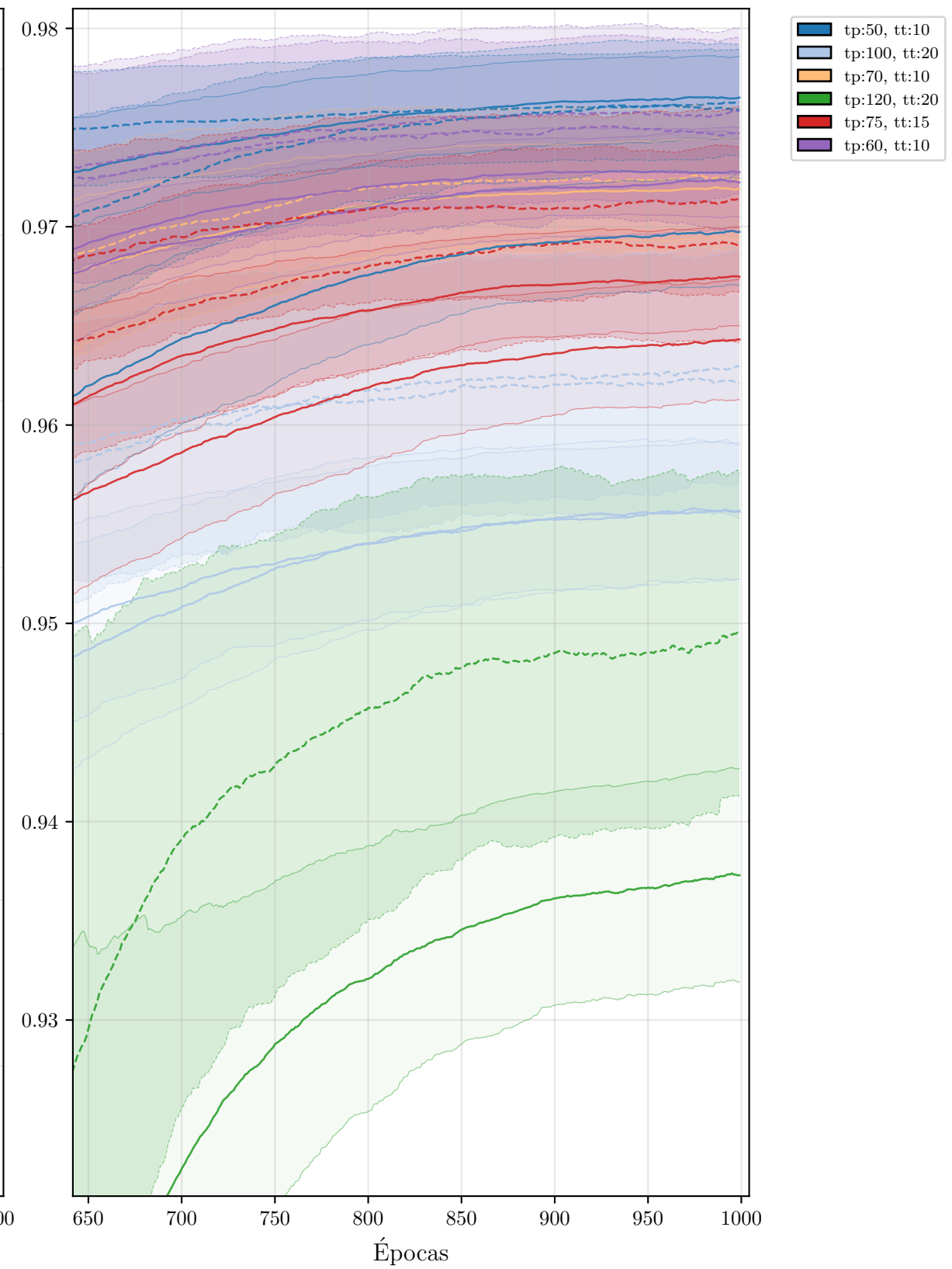
AUC-ROC
