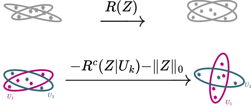
Figura 1.4: Iteración dos pasos do \text{MCR}^2
