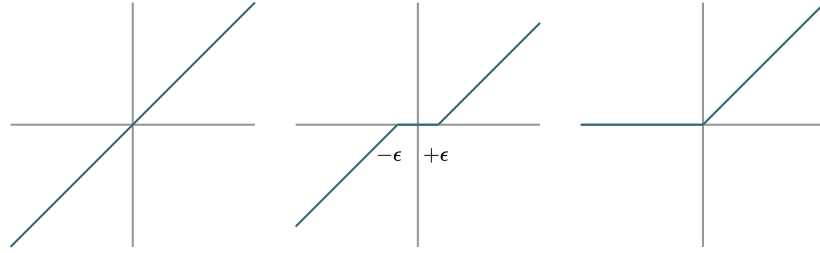
Figura 1.1: Funcións de activación usadas no traballo. (esquerda) Función identidade (centro) Función de umbral suave \sigma_{\epsilon}(\cdot) , parametrizada por \epsilon (dereita) Función ReLU, nótase que a función \sigma_{\epsilon}(x) é indentica (no dominio \mathbb{R}^+ ) a \text{ReLU}(x - \epsilon) .
