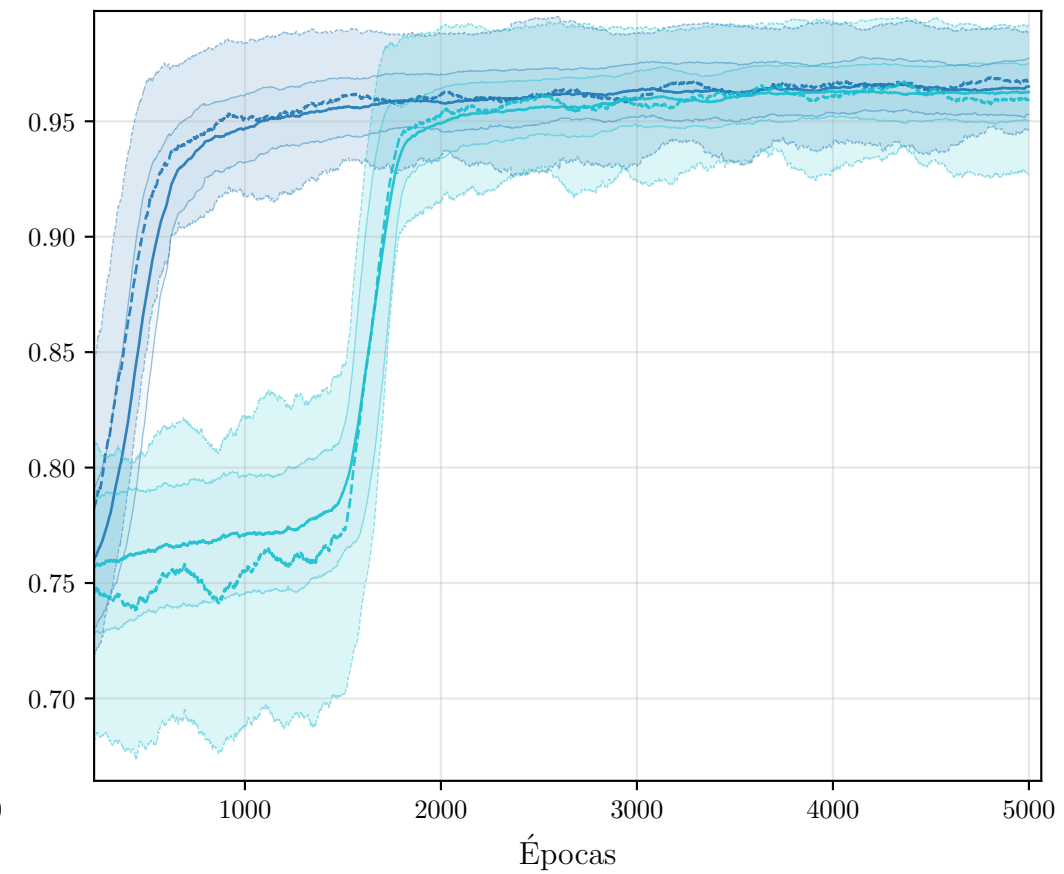
AUC-ROC
