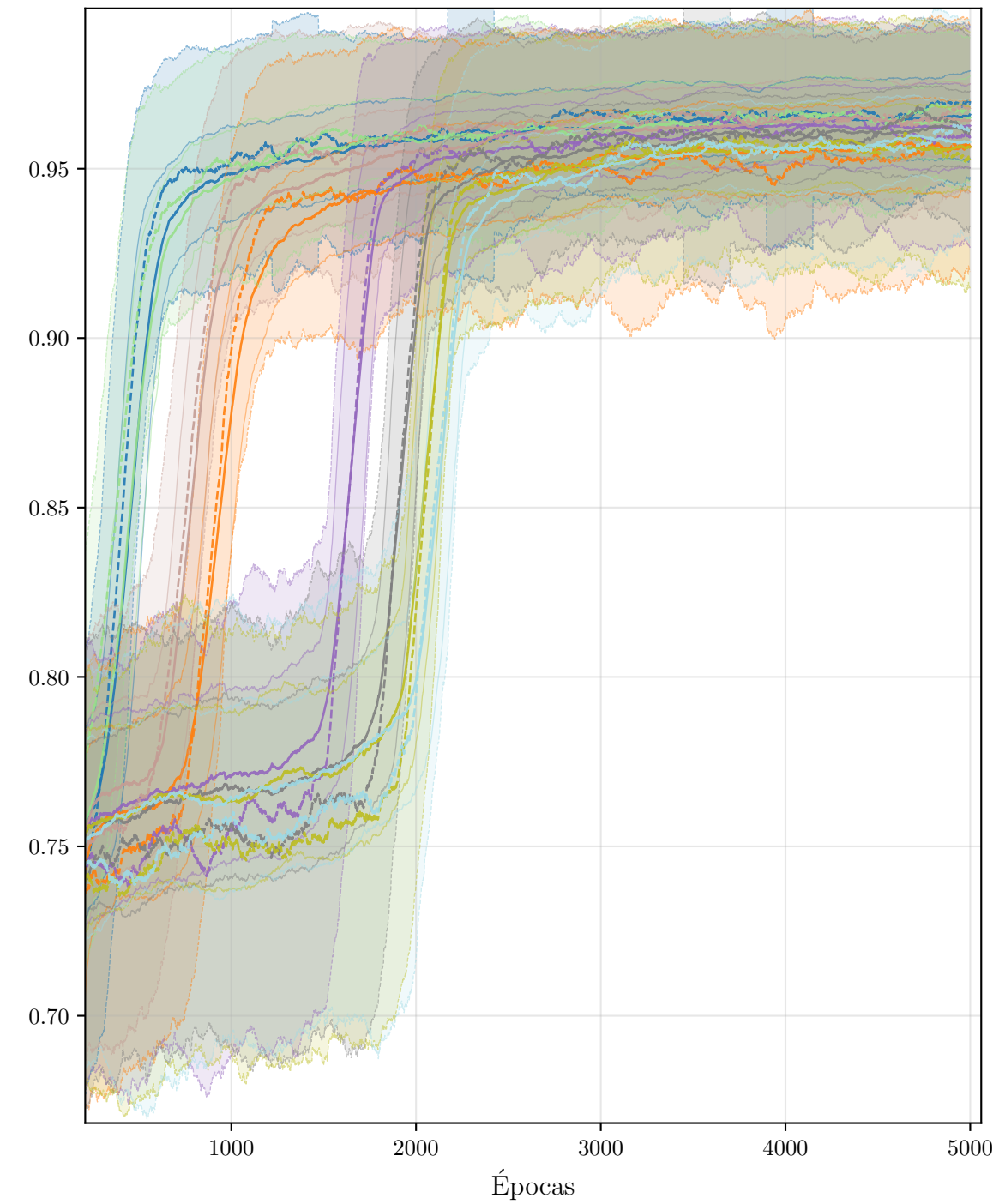
AUC-ROC
