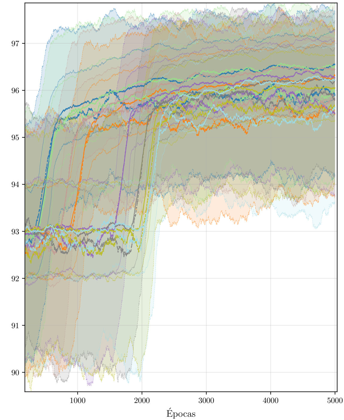
Precisión
