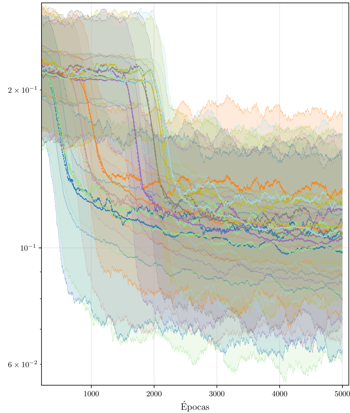
Pérdida
