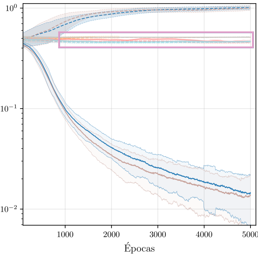
Pérdida
