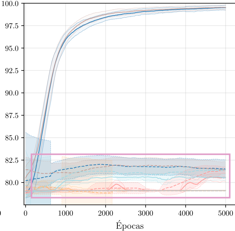
Precisión
