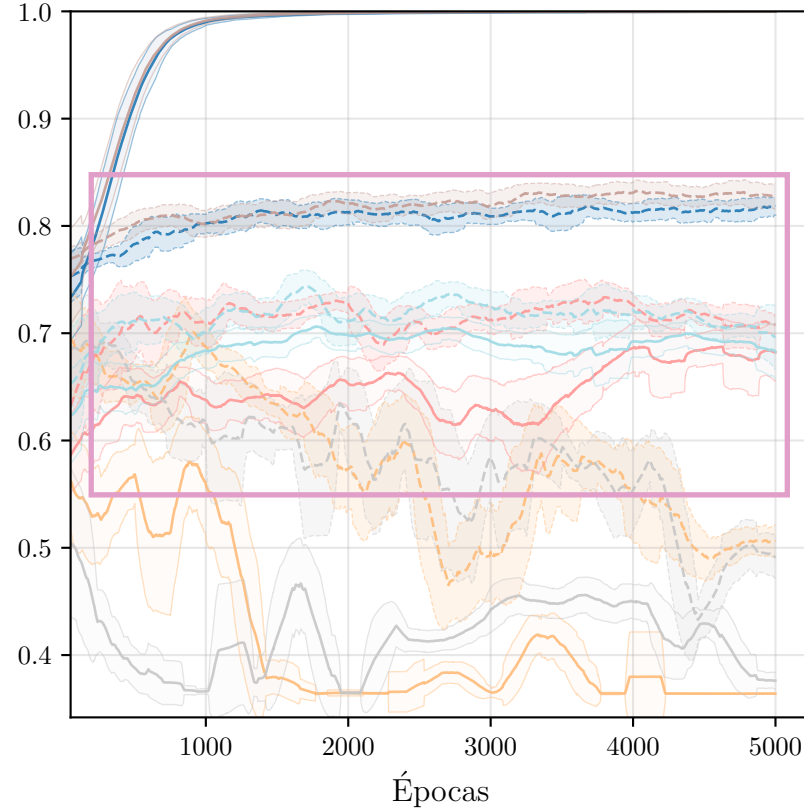
AUC-ROC
