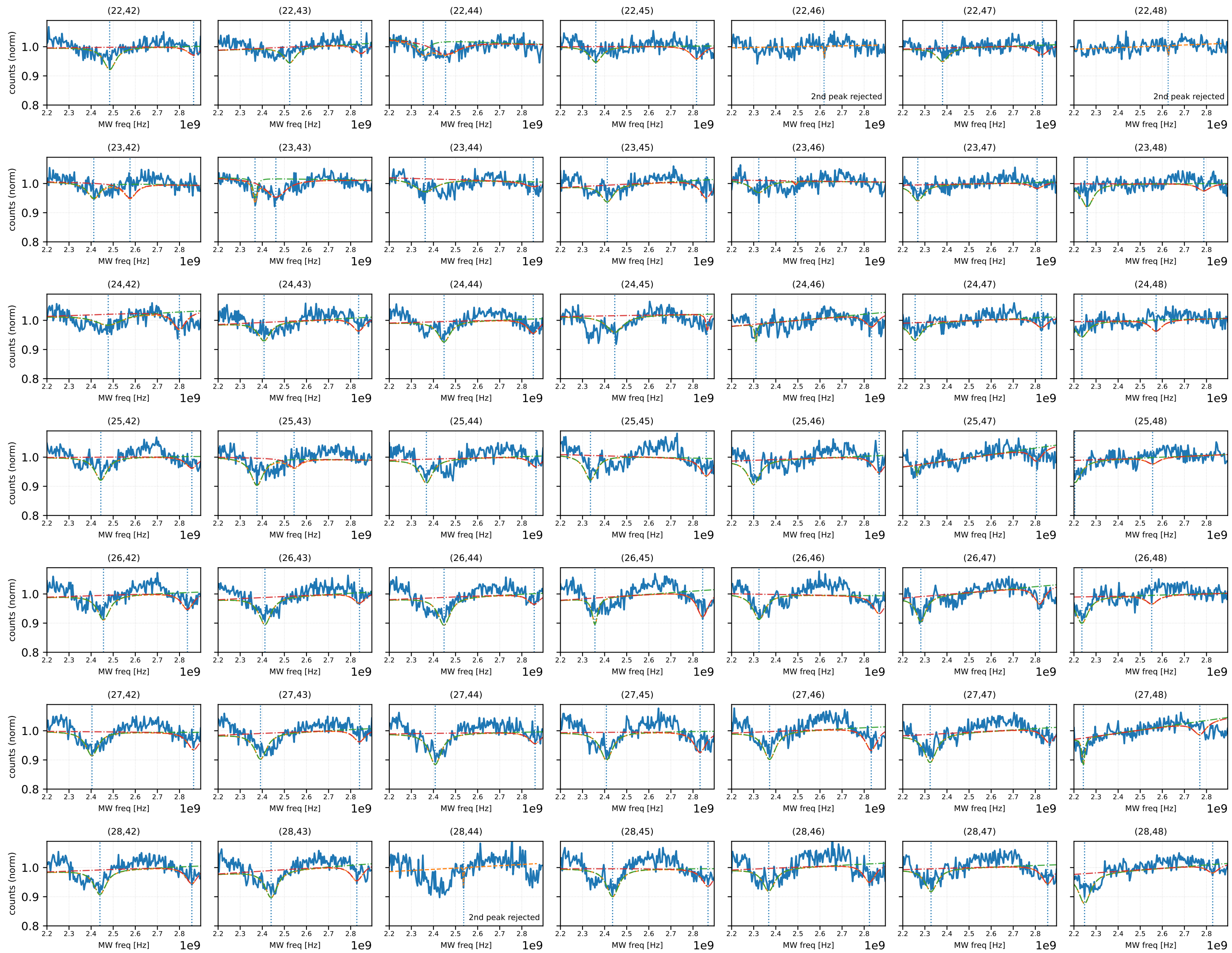
ODMR sweeps — grille autour de (25,45) | fit: lorentz | thr=20%
