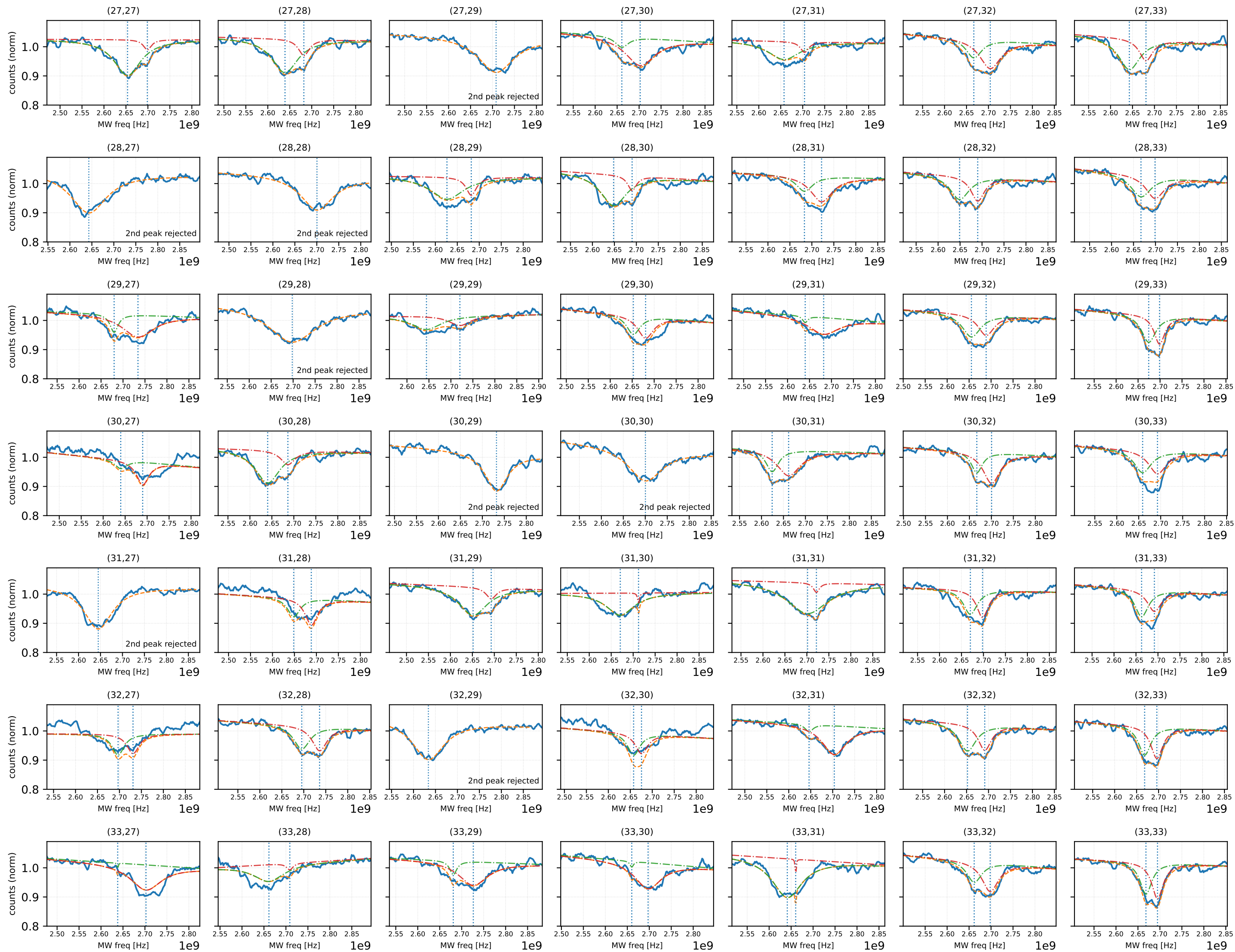
ODMR sweeps — grille autour de (30,30) | fit: lorentz | thr=20%
