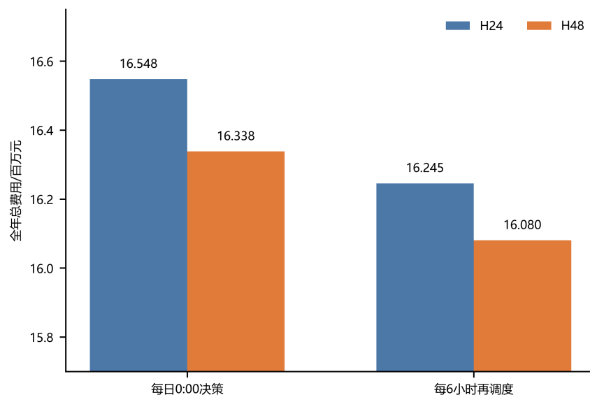
图 14 波动电价下每日决策与 6 小时再调度的全年总费用
