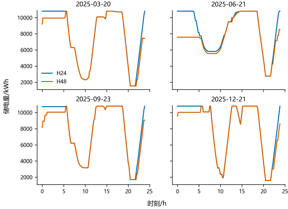
图 13 4 个指定日期的 H24 与 H48 实际储能轨迹
