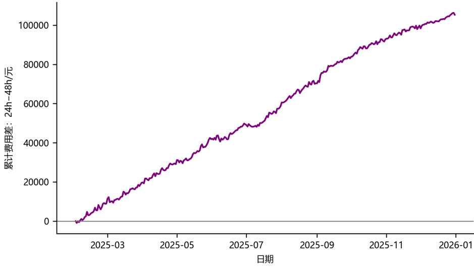
图 12 全年累计费用差 \sum_d (C_d^{H24} - C_d^{H48})
