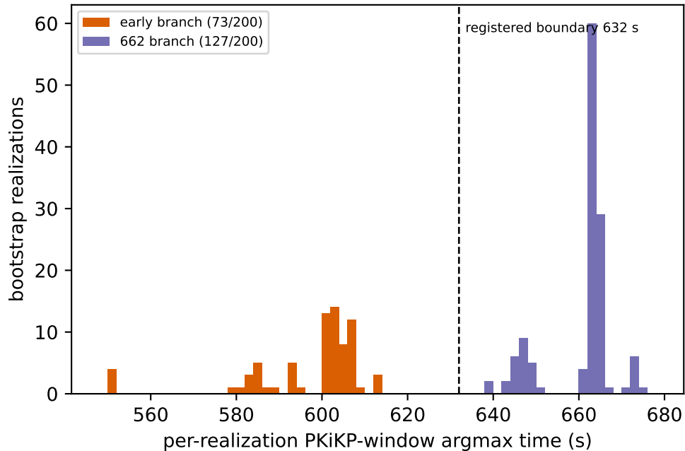
Type I bootstrap argmax times (methods_robustness_200)
