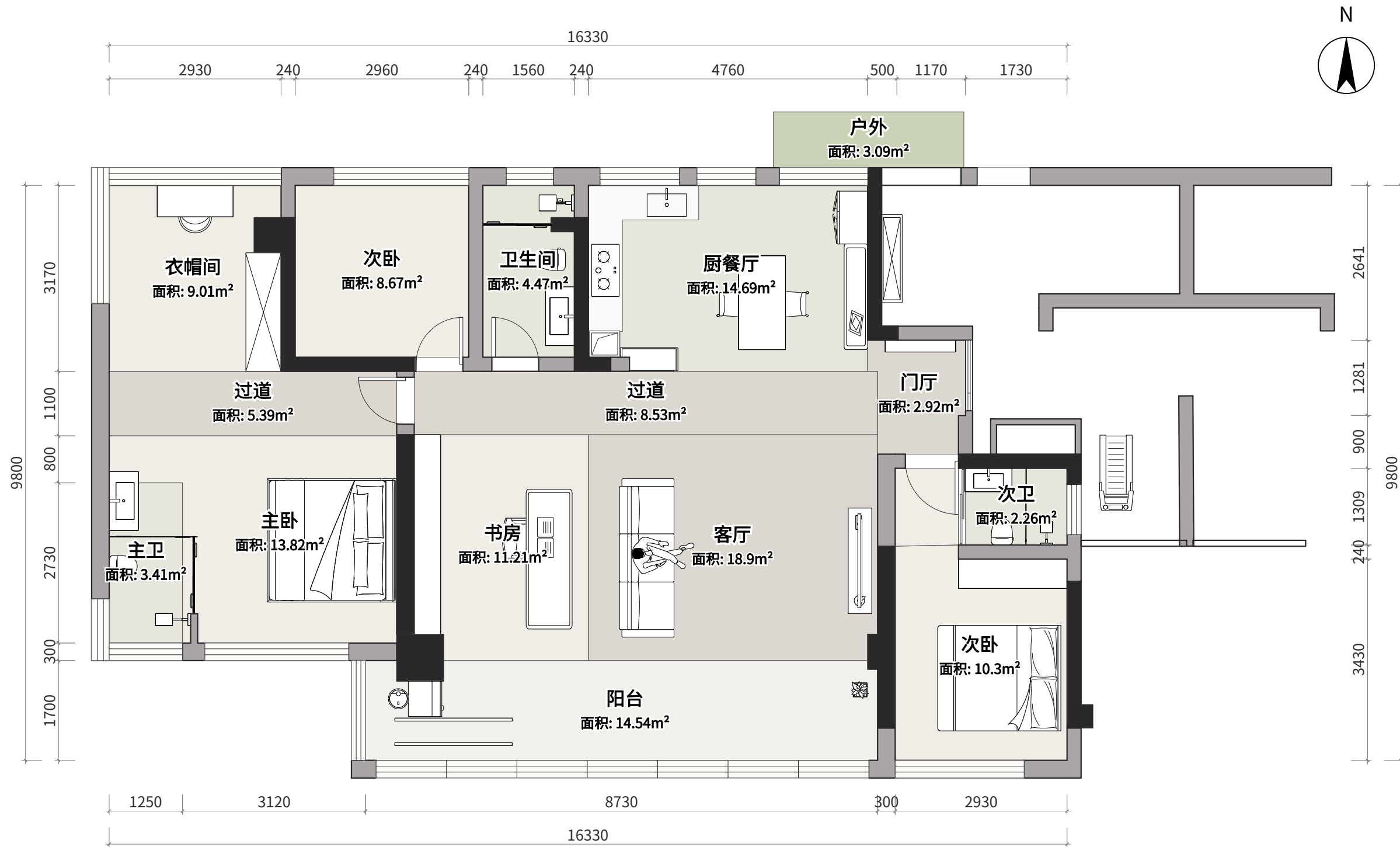
兰亭序 - 基础 - 平面图 套内面积: 131.51m 2
