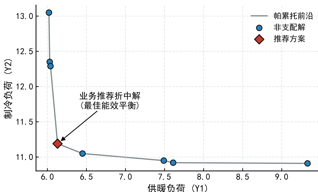
图 5-2 帕累托前沿
