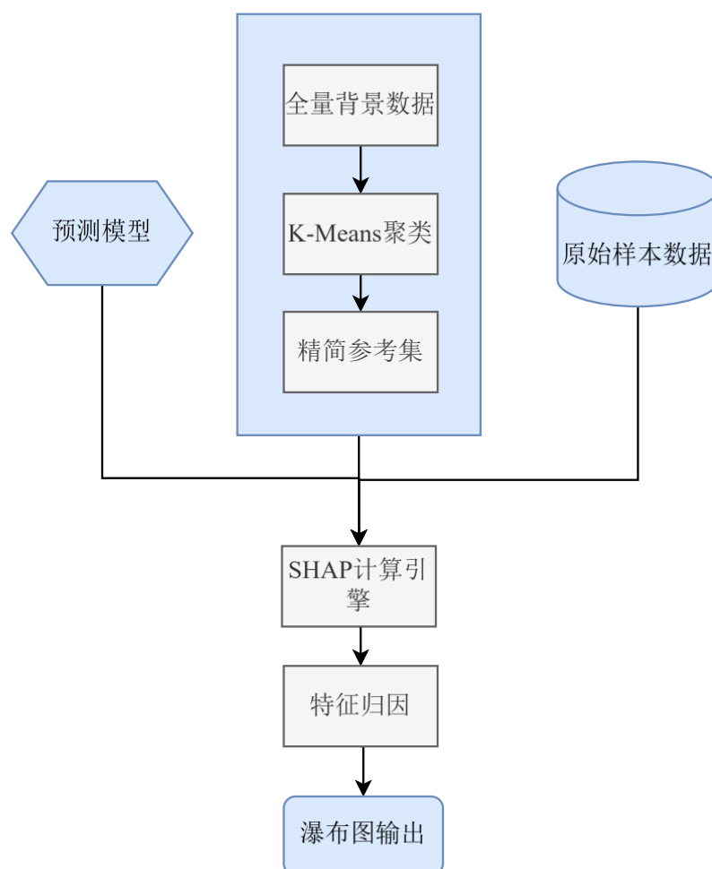
图 4-1 SHAP 流程图
