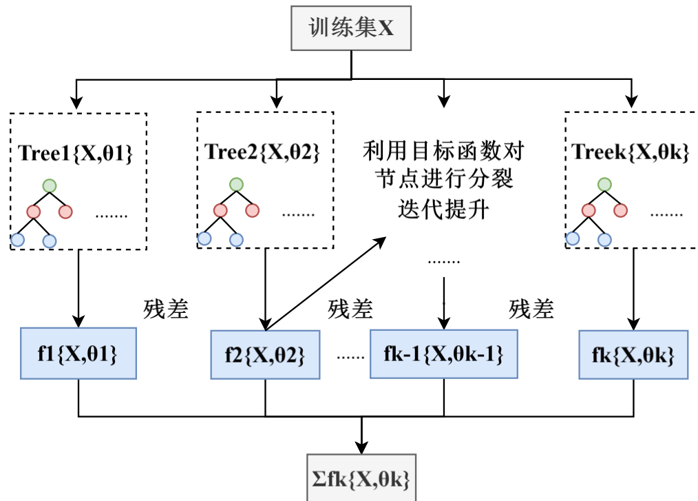
图 3-2 XGBoost 架构图
