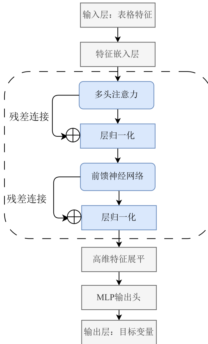
图 3-4 Tabular Transformer 架构图
