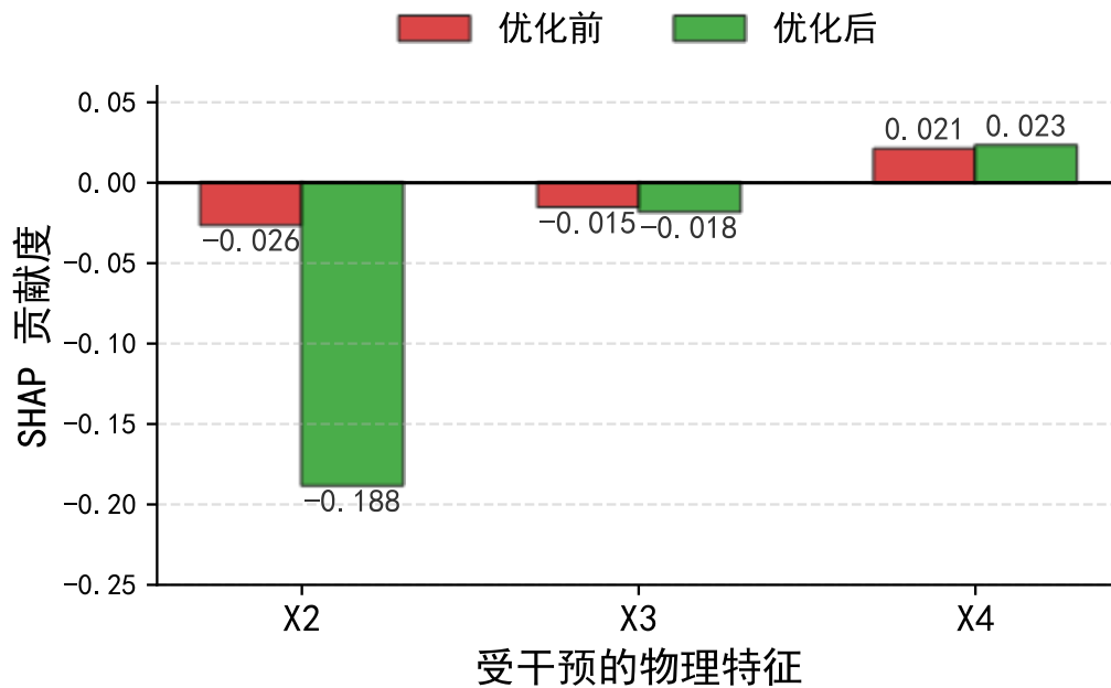
图 4-3 贡献度对比图
