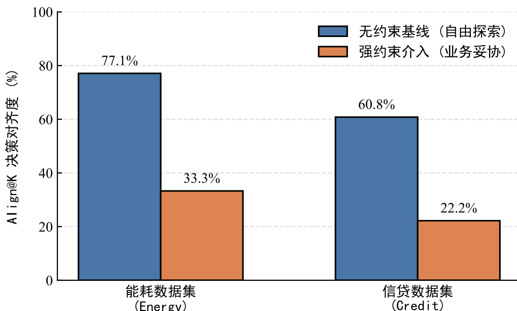
图 6-1 决策对齐度指标
