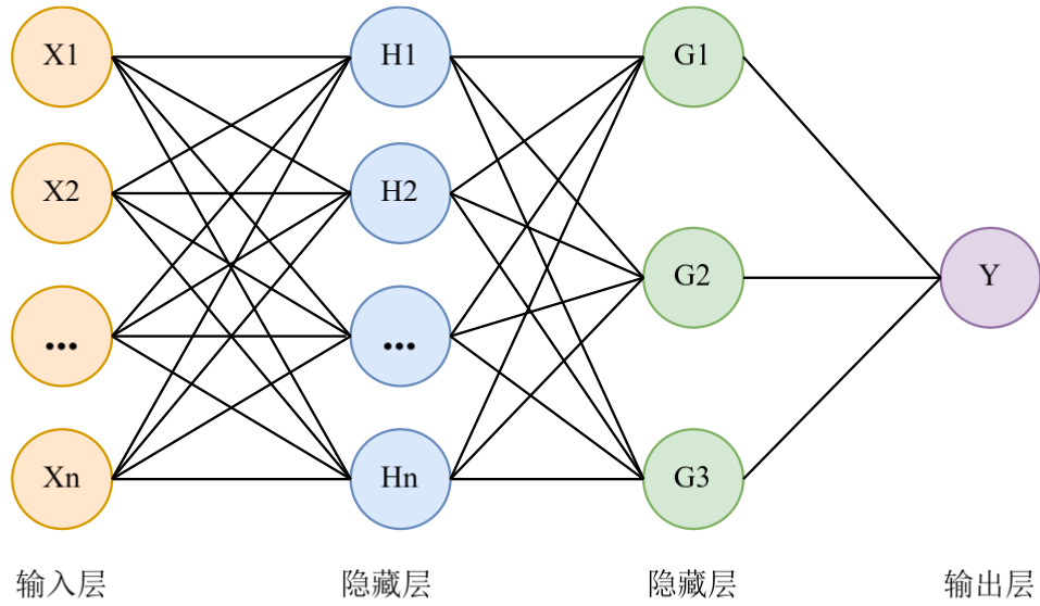
图 3-3 MLP 架构图
