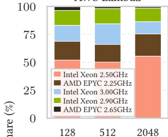
AWS Lambda
