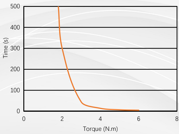
堵转工况最大过载曲线 (Max Overload)
