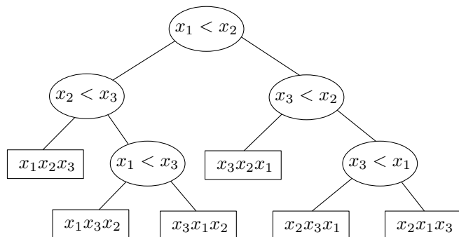
Obrázek 3.1: Příklad rozhodovacího stromu pro 3 různé prvky
