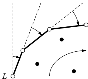
Obrázek 16.2: Provázkový algoritmus
