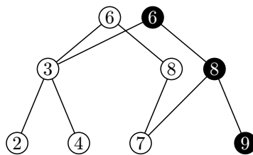
Obrázek 16.12: Vložení prvku 9 do persistentního stromu
