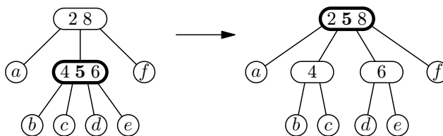
Obrázek 8.8: Štěpení přeplněného vrcholu při vkládání do (2, 3) -stromu
