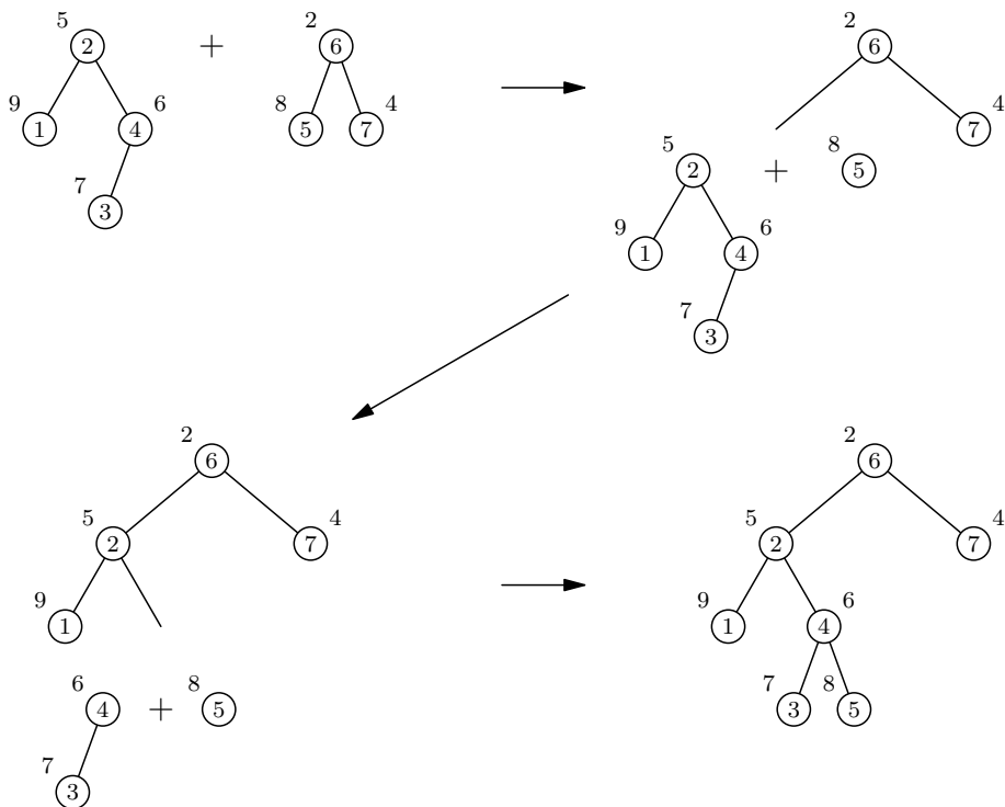
Obrázek 11.4: Spojení dvou treapů.
