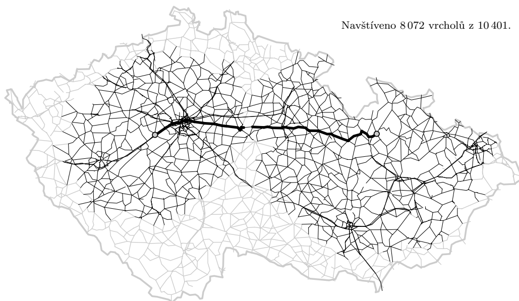
Obrázek 6.4: Hledání v mapě obousměrným Dijkstrovým algoritmem
