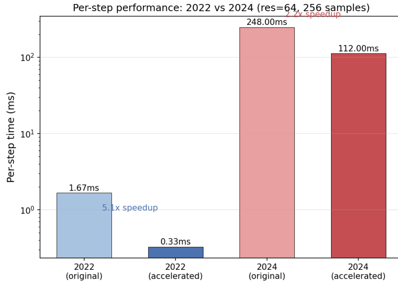
Figure 3: 单步耗时柱状图（ 64 \times 64 ，256 采样）：2022 加速后 0.33 ms/步，2024 加速后 112 ms/步。2022 快约 341 倍。
