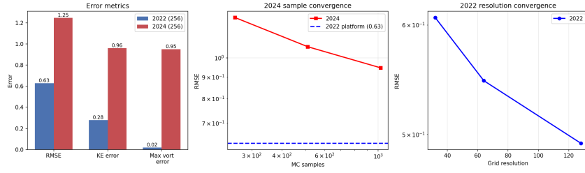
Figure 6: 定量误差分析：左——主要误差指标对比；中——2024 误差随采样数的收敛（虚线为 2022 平台值）；右——2022 误差随网格分辨率的收敛。
