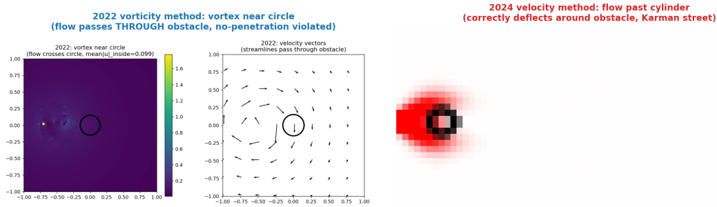
Figure 7: 复杂边界对比：左——2022 涡量法在涡旋靠近圆形障碍物时的速度场（流线直接穿过障碍物，违反不可穿透边界）；右——2024 速度法正确使流动绕开圆柱，产生 Kármán 涡街。
