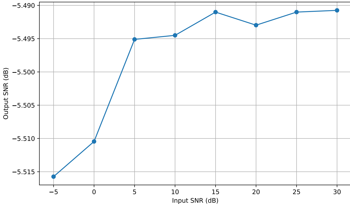
Output SNR vs Input SNR — AM TRF
