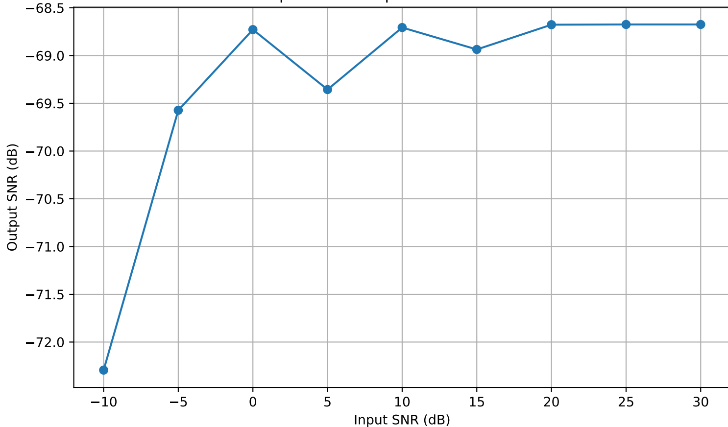
Output SNR vs Input SNR — NBFM TRF
