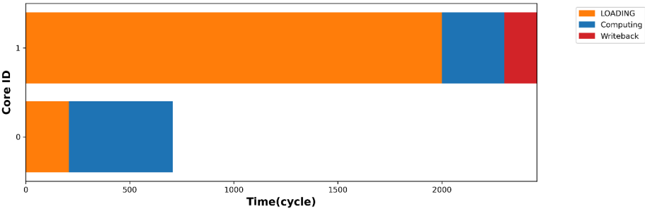
图 5-1 MB-1 状态转移时间线 (全后端。数据见附录附录 A.5)。横轴为仿真周期 (cycle), 纵轴为两核 (上方为 Core 1, 下方为 Core 0)。图中颜色表示各核所处状态: 橙色为 Loading, 蓝色为 Computing, 红色为 Writeback
