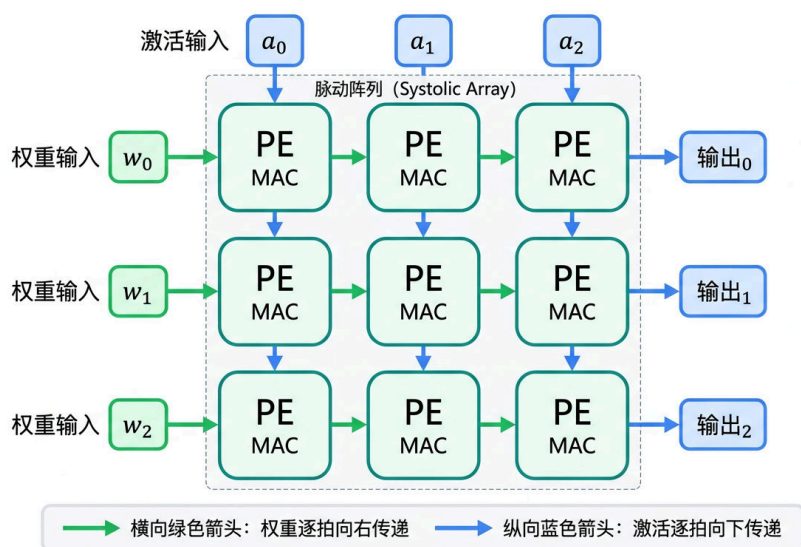
图 2-3 3×3 脉动阵列数据流示意图
