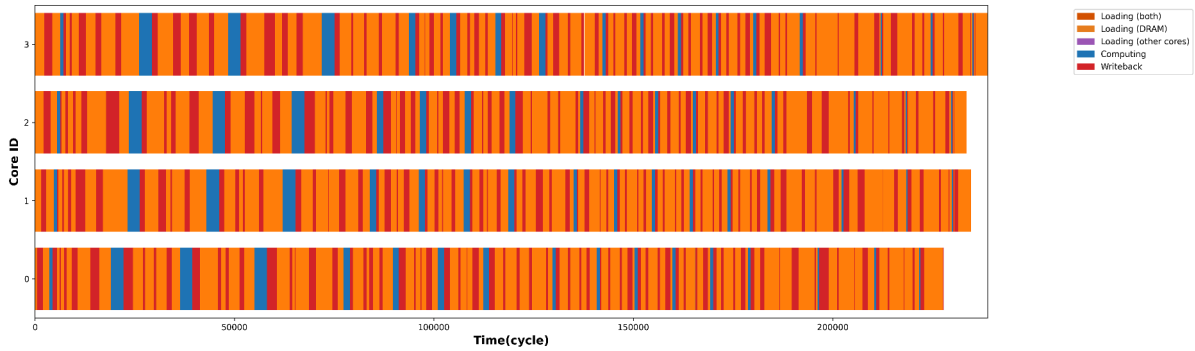
图 5-5 DDR4 基线甘特图 ( 2 \times 2 , ResNet50 批 1)。橙色为加载（含 DRAM 与核间等待），蓝色为计算，红色为写回。加载阶段占据大部分时间线
