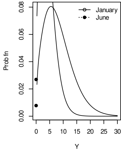
Tweedie distribution
