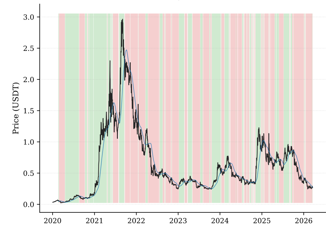
ADA/USDT
