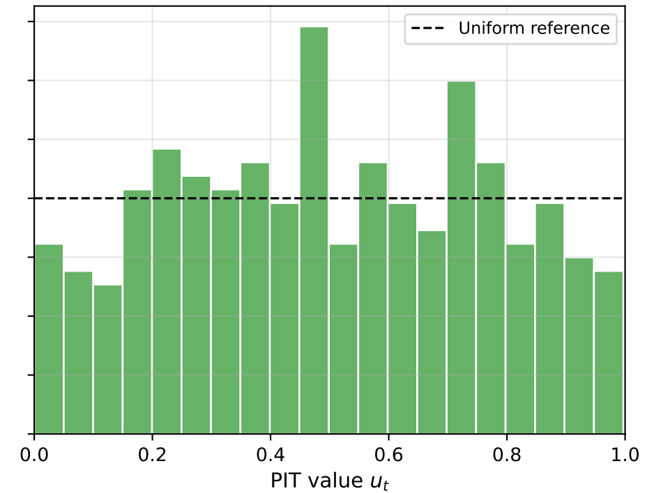
GARCH(1,1)
