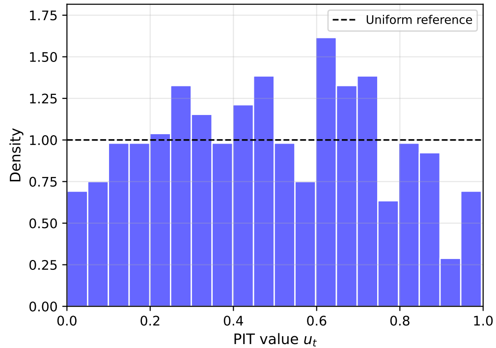
NLL LSTM
