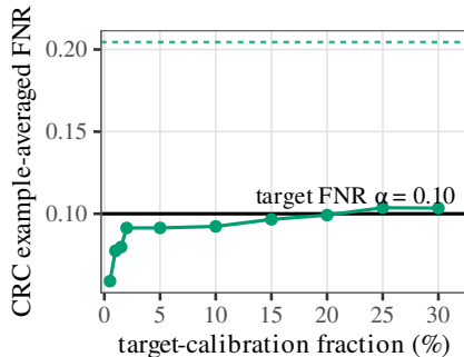
BigEarthNet-S2 ( \alpha = 0.10 )
