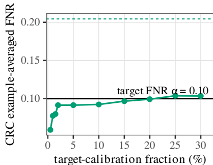
BigEarthNet-S2 ( \alpha = 0.10 )
