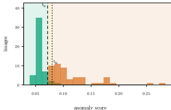
(d) VisA pcb1 / dinomaly G1 + G2 certified
