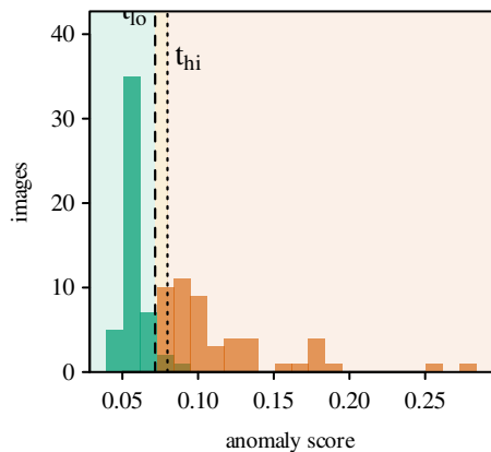
(d) VisA pcb1 / dinomaly G1 + G2 certified
