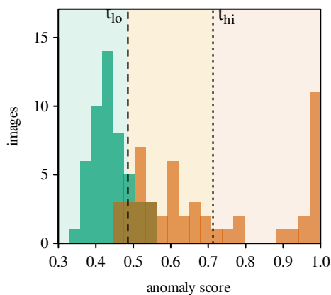
(d) VisA pcb1 / dinomaly G1 + G2 certified
