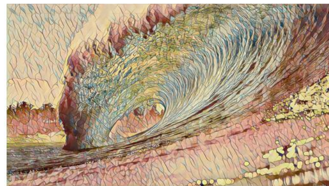
FaintManga
