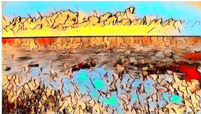
Starry Night (150%)
