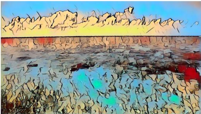
Starry Night (100%)
