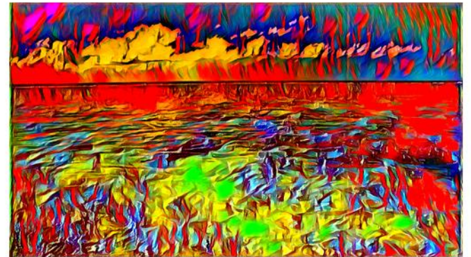
Hundertwasser (200%)
