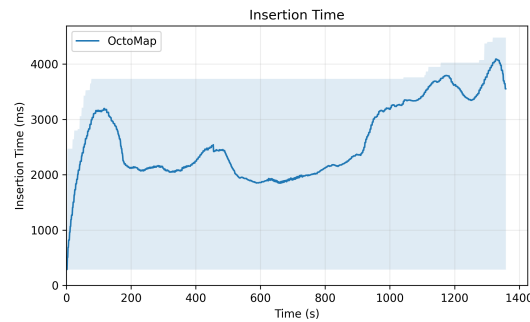
(d) Point cloud insertion time over the duration of dataset experiment 0402
