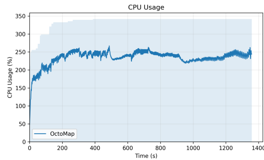
(d) CPU usage over the duration of dataset experiment 0402
