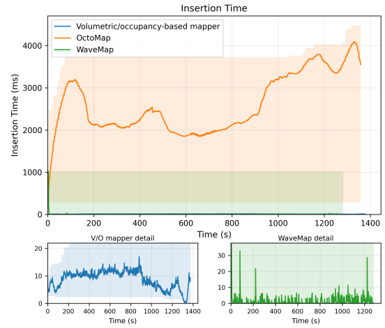
(d) Point cloud insertion time over the duration of dataset experiment 0402
