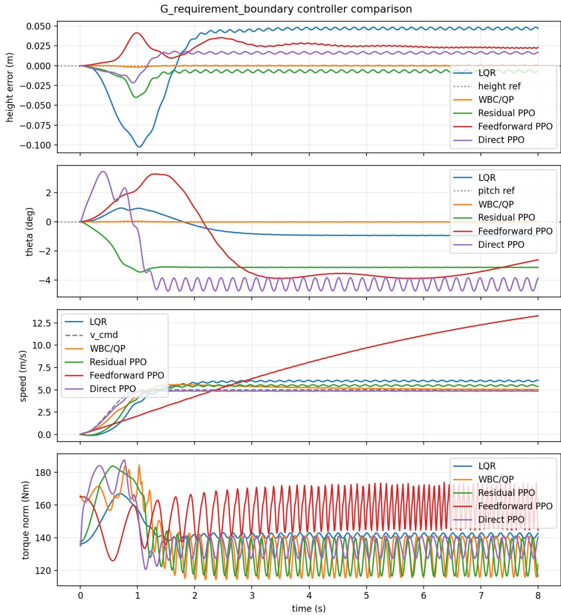
图 15: 场景 G 中五种控制器的叠加对比。
