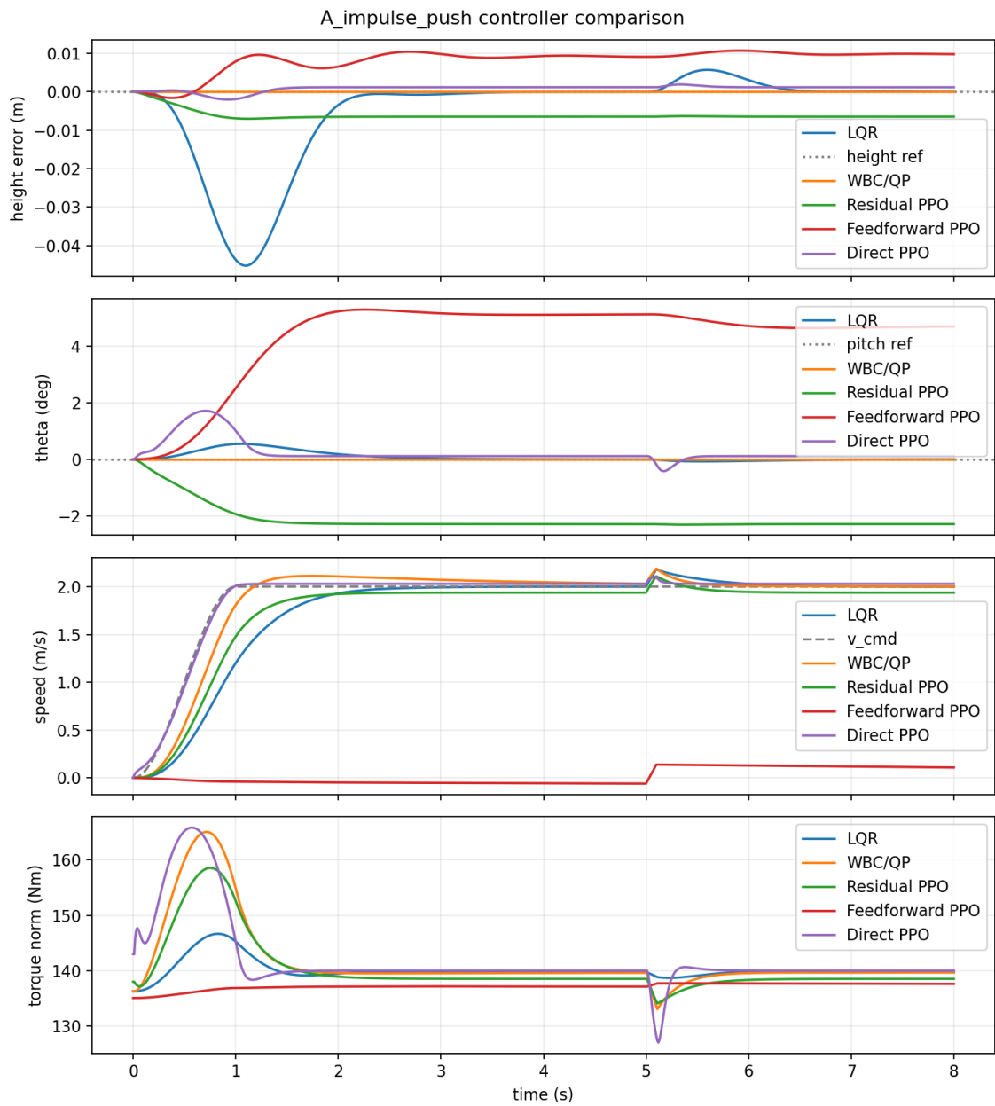
图 2: 场景 A 中五种控制器的叠加对比。
