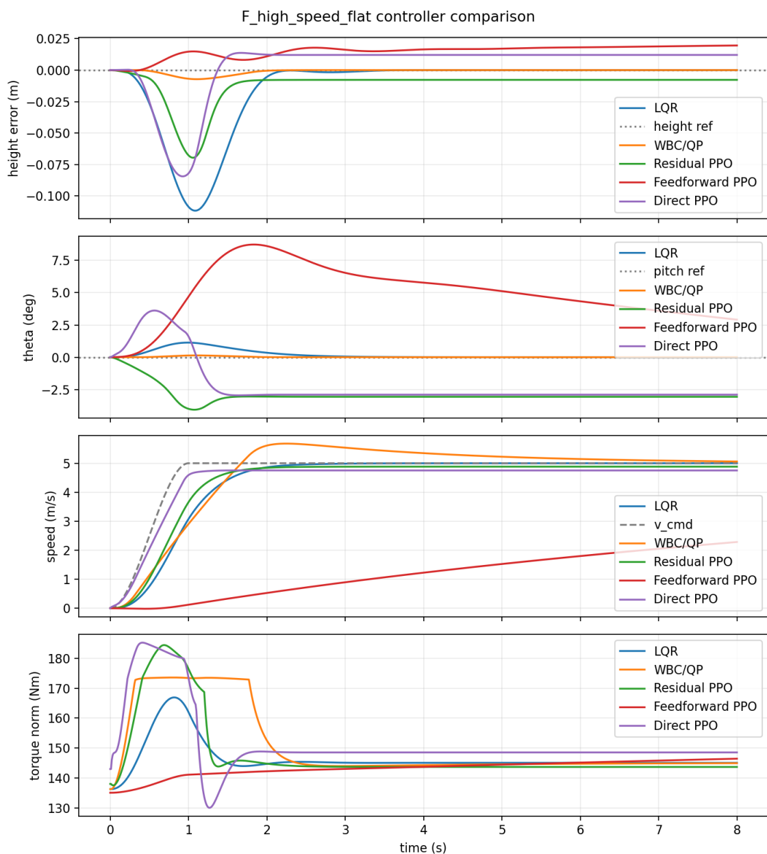
图 14: 场景 F 中五种控制器的叠加对比。
