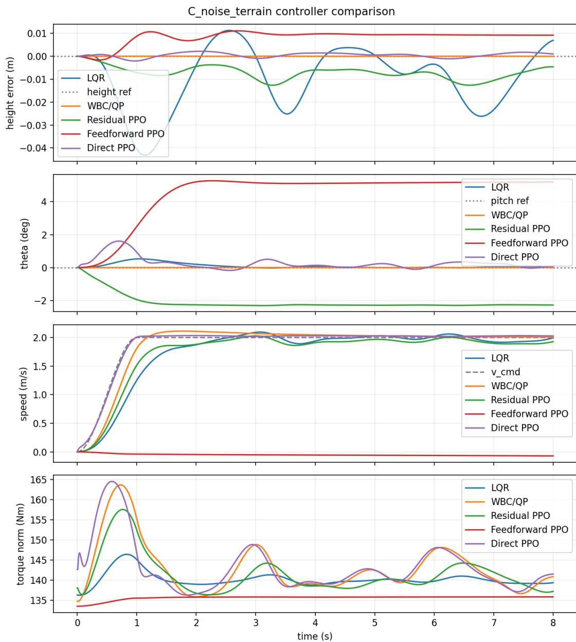
图 8: 场景 C2 中五种控制器的叠加对比。
