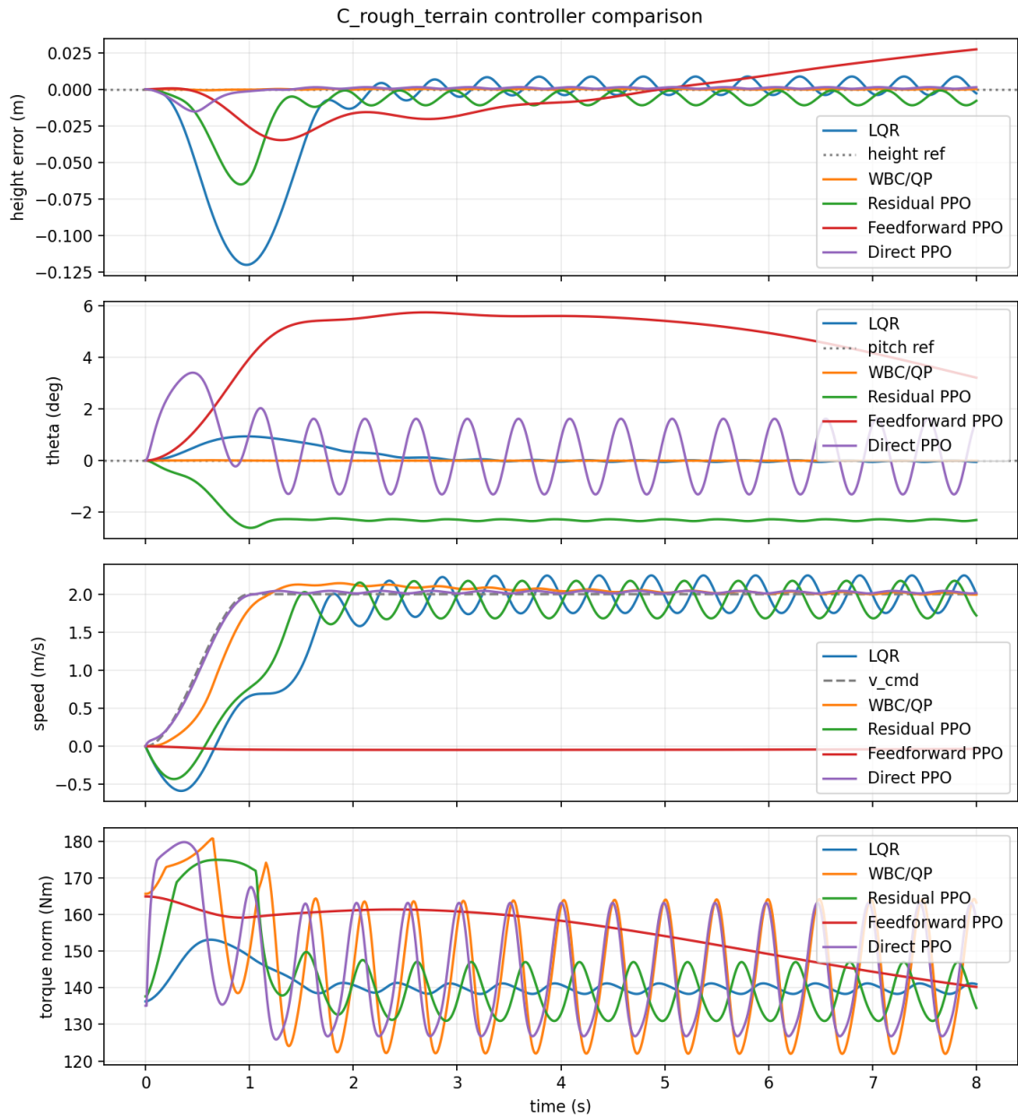
图 6: 场景 C1 中五种控制器的叠加对比。
