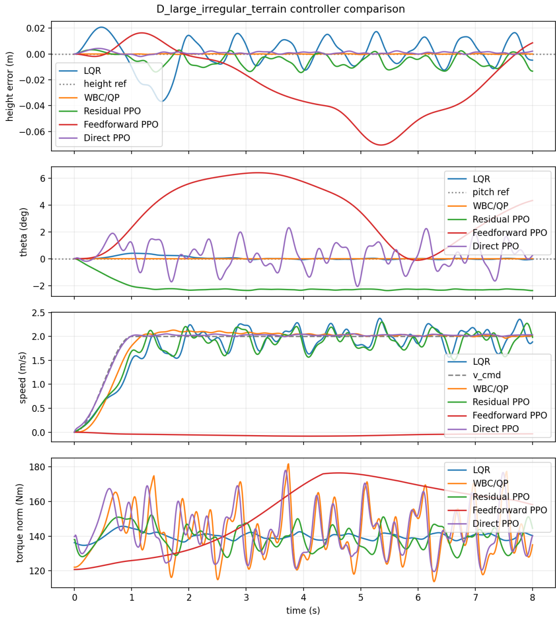
图 9: 场景 D 中五种控制器的叠加对比。
