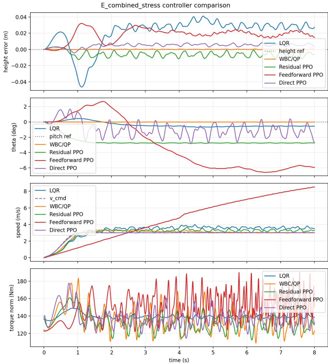
图 11: 场景 E 中五种控制器的叠加对比。
