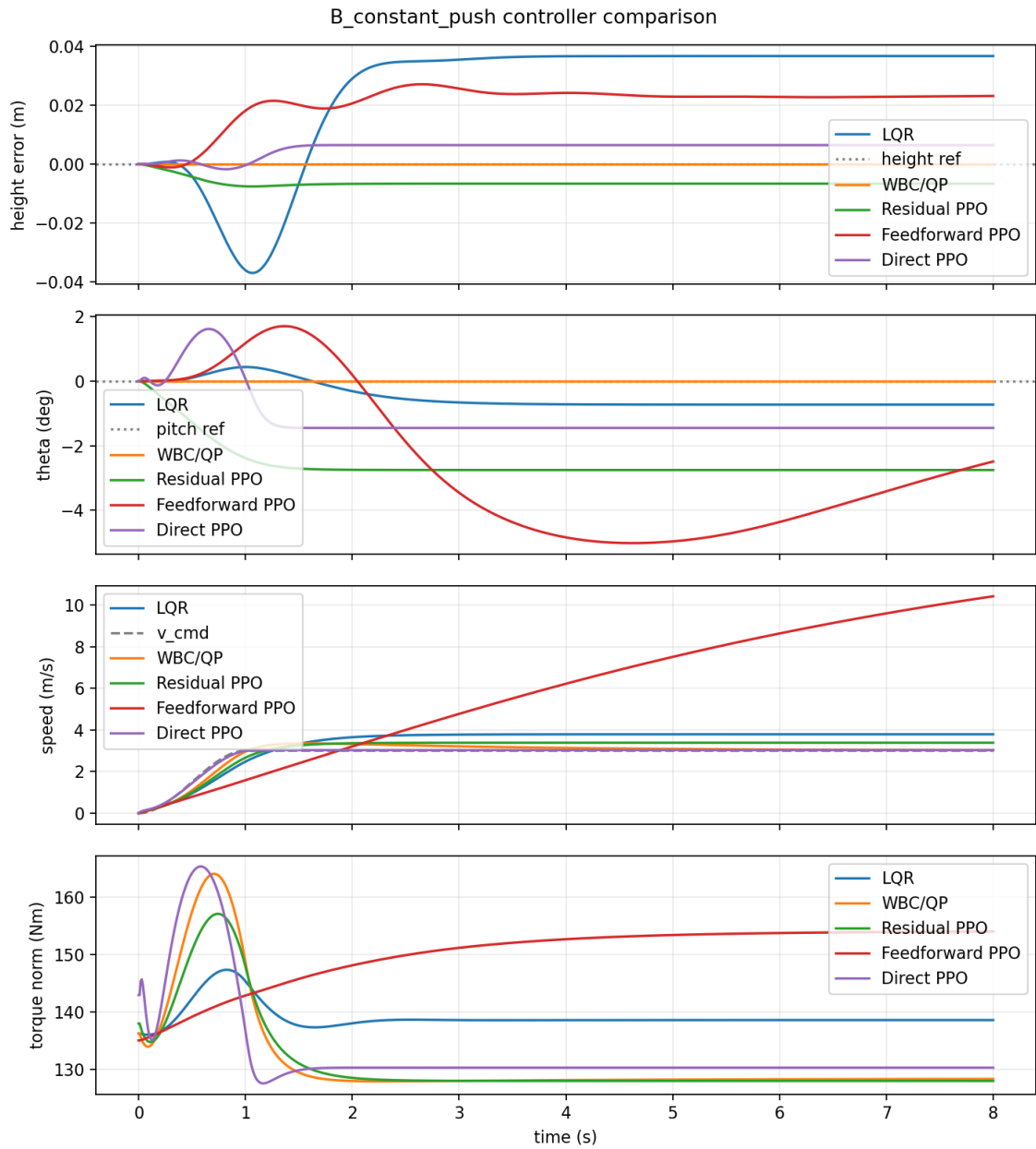
图 4: 场景 B 中五种控制器的叠加对比。
