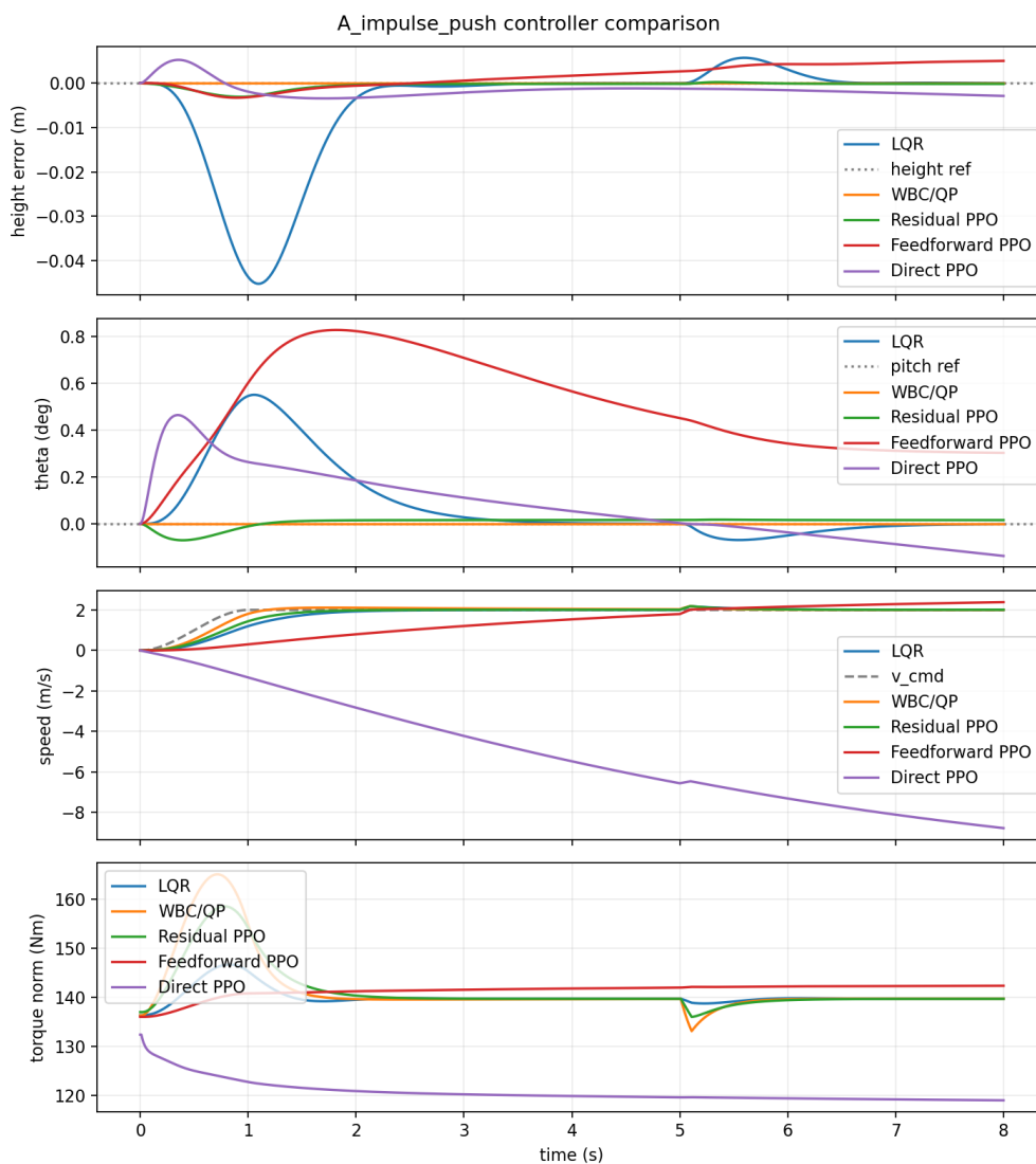
图 3: 场景 A 的五控制器叠加曲线。冲击发生在 t = 5 s；启动阶段对高度和速度误差的贡献大于短脉冲本身。
